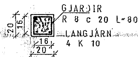
SÚLA S.1.4. 1:20
