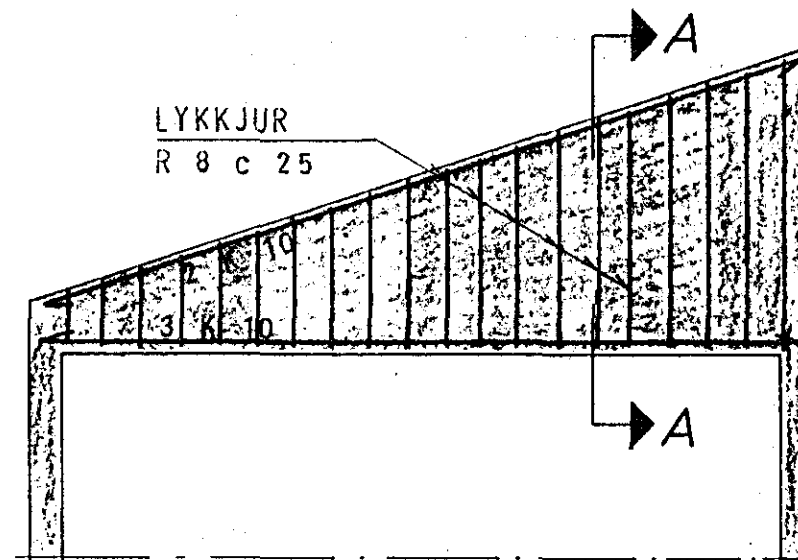
BITI B.12. 1:50
