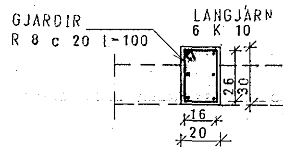
SÚLA S.1.1. 1:20
