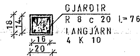
SÚLA S.1.2. 1:20
