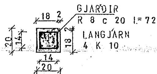
SÚLA S.1.3. 1:20
