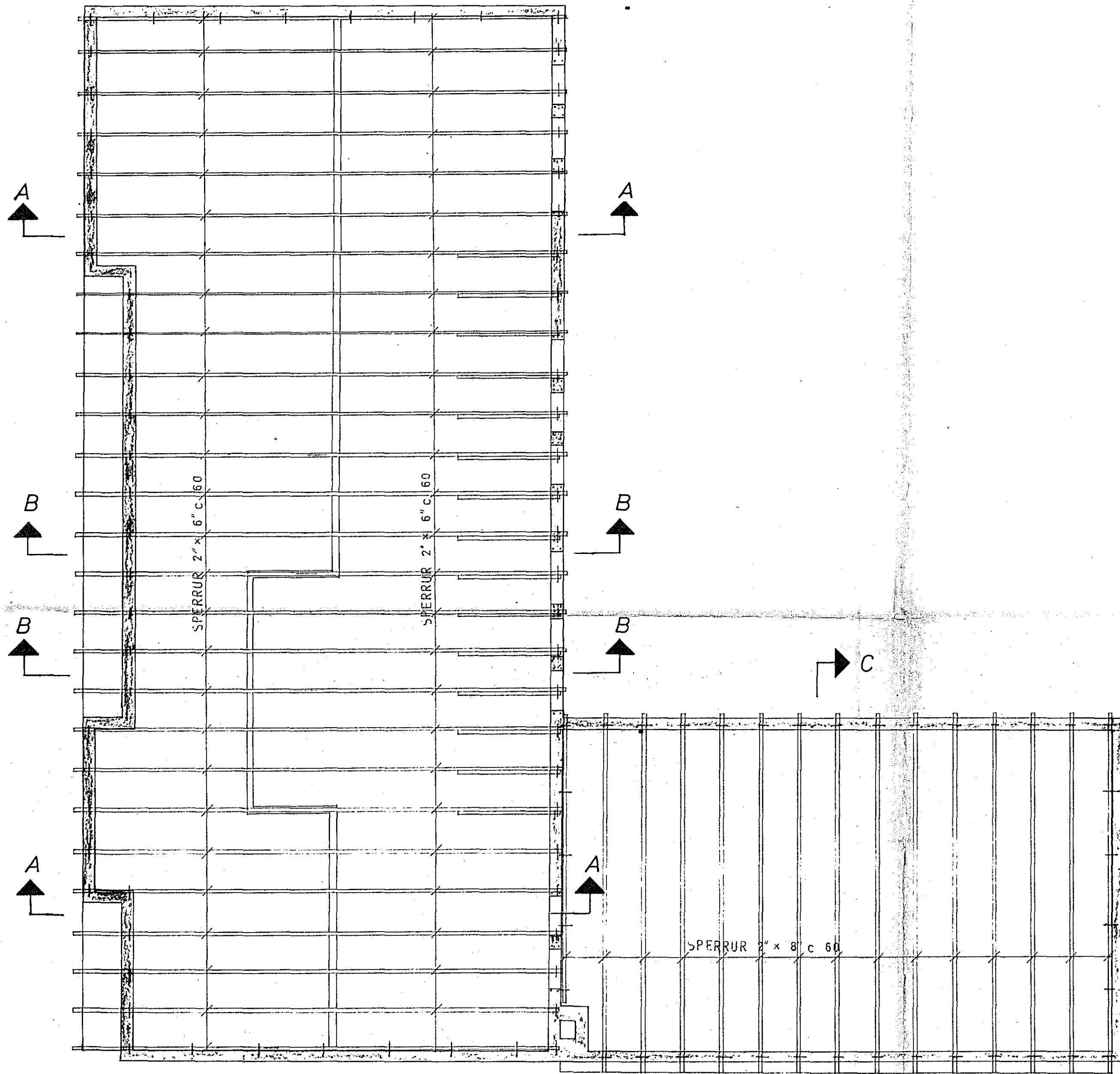
GRUNNMYND - RIS 1:50
