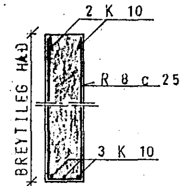
SNID A-A 1:20
