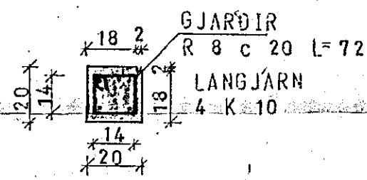
SÚLA S.1.3. 1:20
