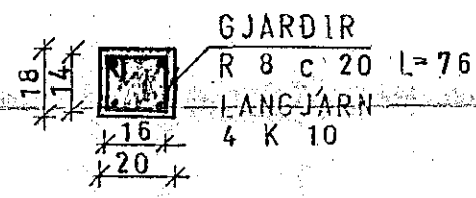
SÚLA S.1.2. 1:20
