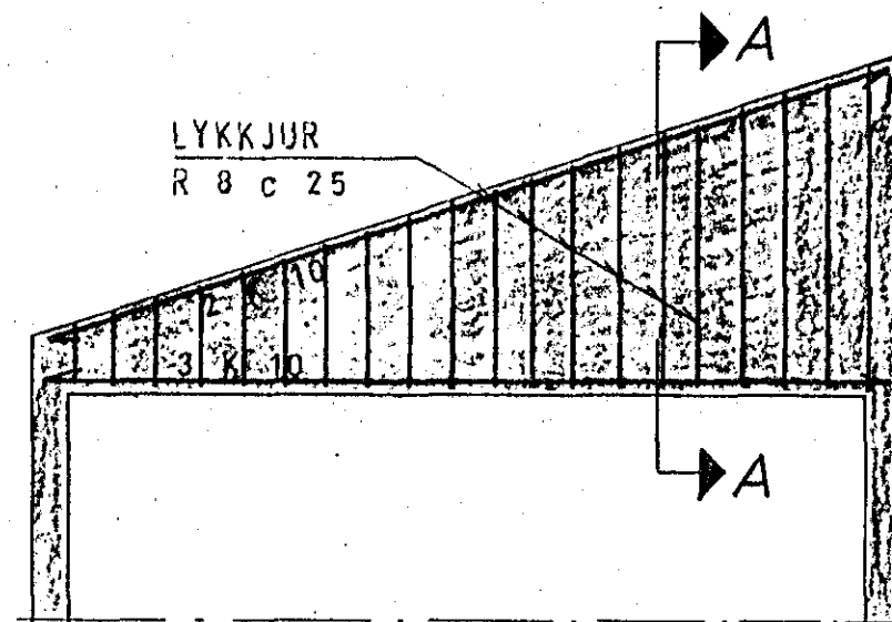
BITI B.12. 1:50
