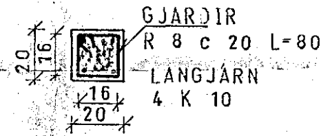
SÚLA S.1.4. 1:20
