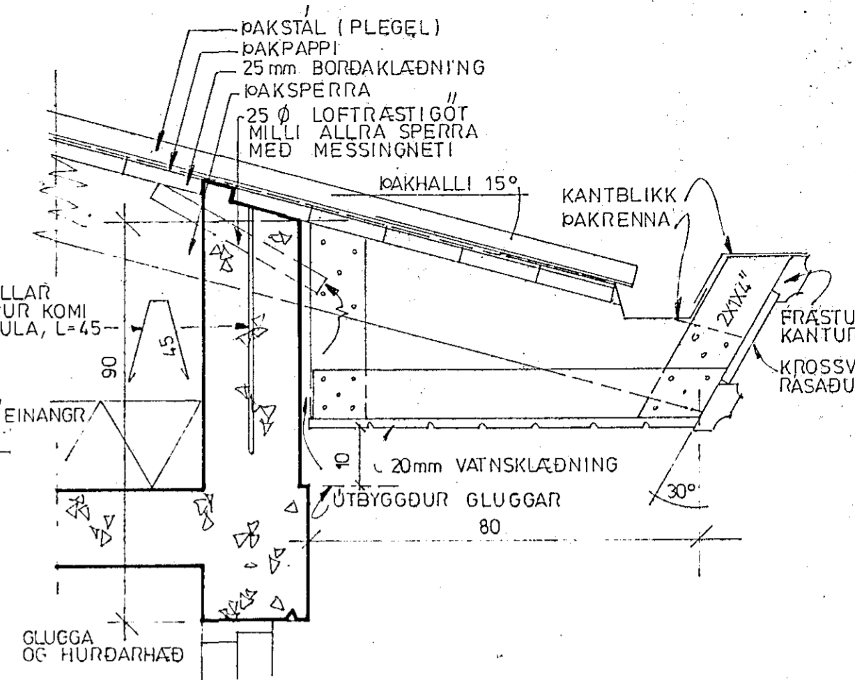
SNID A- (FRÁGANGUR VIÐ ÞAKKANT OG ÞAK.)
