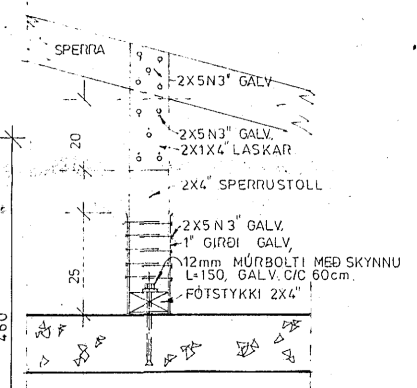
SNID B- (FRÁGANGUR A STÖLUN VIÐ SPERRUR.)
