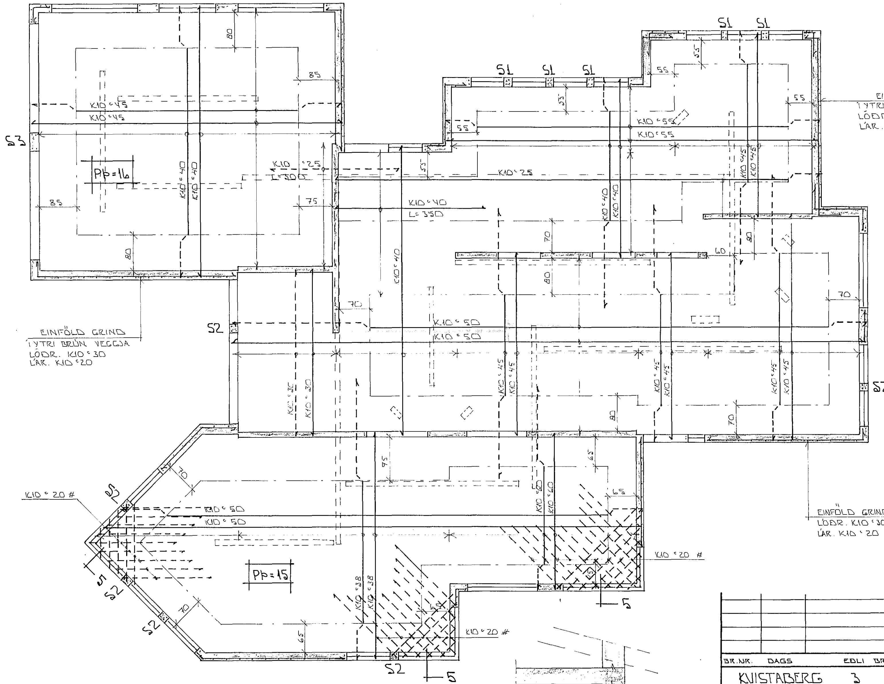
GRUNNMYND 1:50
