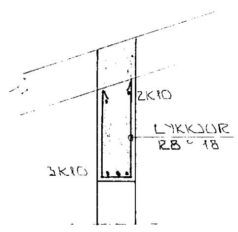
SNID 7 I BITA YFIR BILG. OG GL. 1:20
