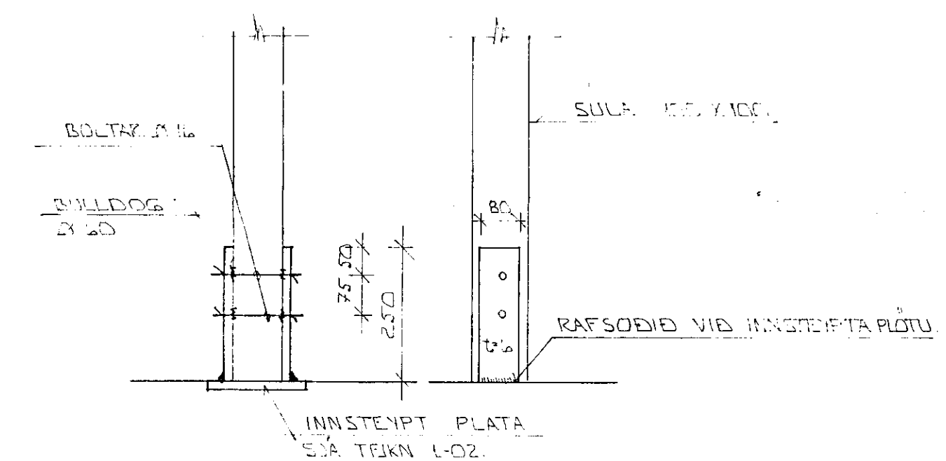
FESTING SÚLU I GÖLF 1:10
