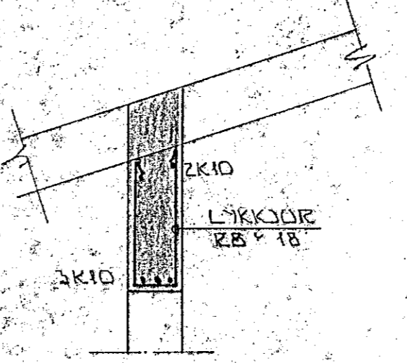
SNID 7 I BITA YFIR BILG. OG GL. 1:20
