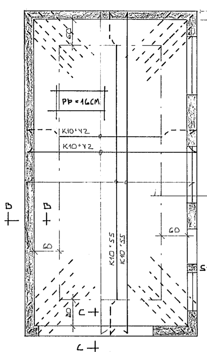
GRUNNMÝND \approx 1:50 JÄRNBENDING PAKPLÖTU.
