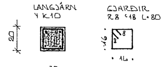
SÚLA S1 \approx 1:20
