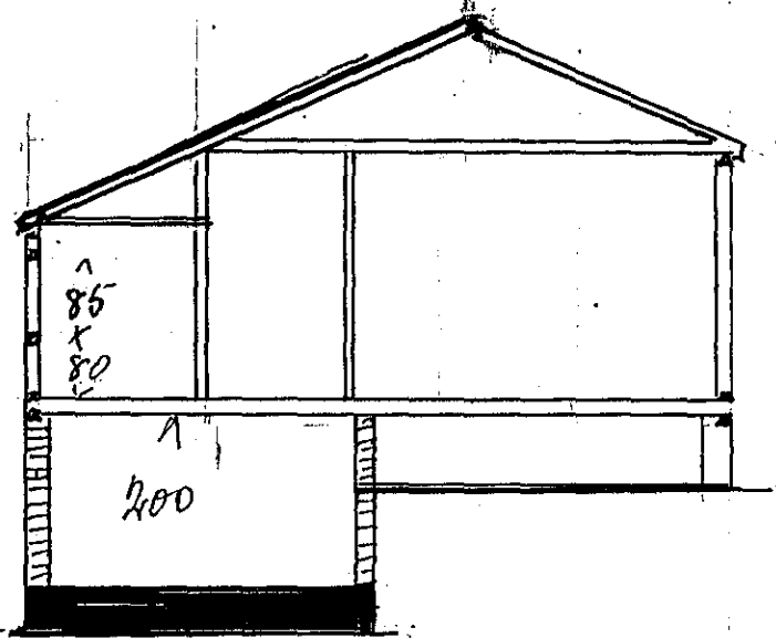
SKURÐUR A-A
