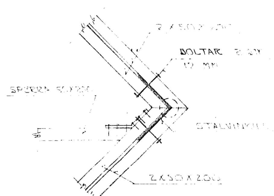
ASIND Y - Y - 1:10
