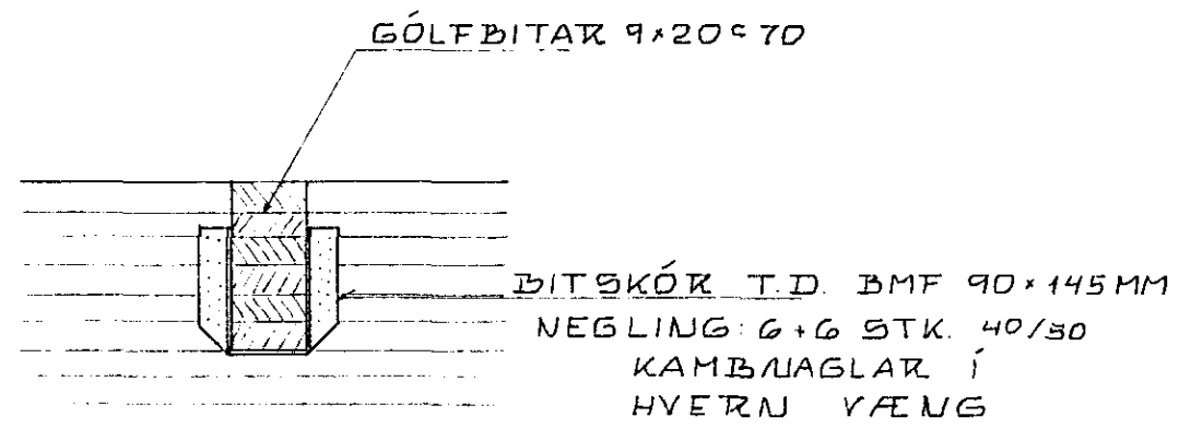
SNIÐ IIa - IIa 1:10
