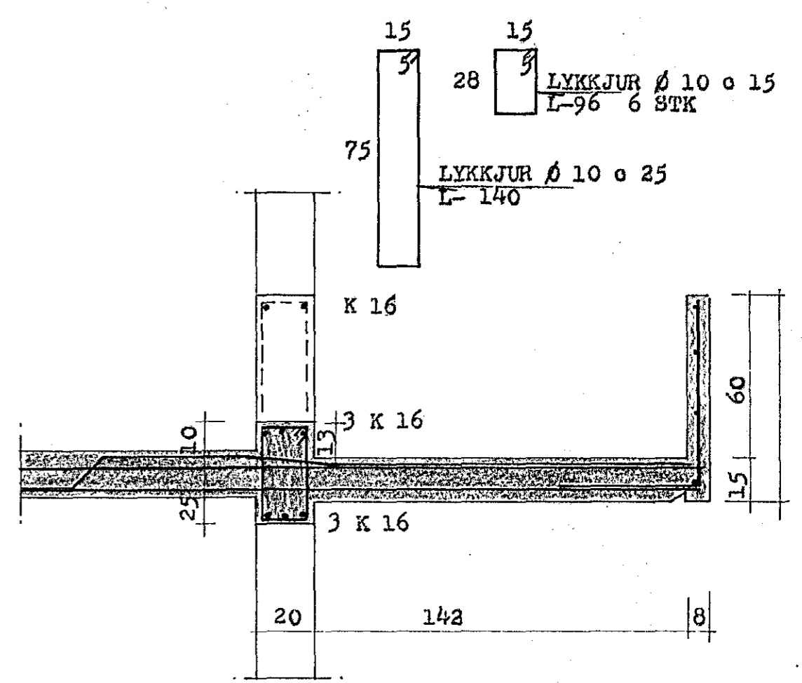
SNID I B-1 1:20
