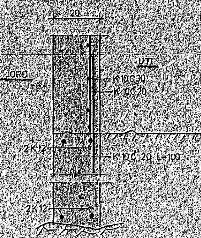
SNÍÐ E-E 1:10
