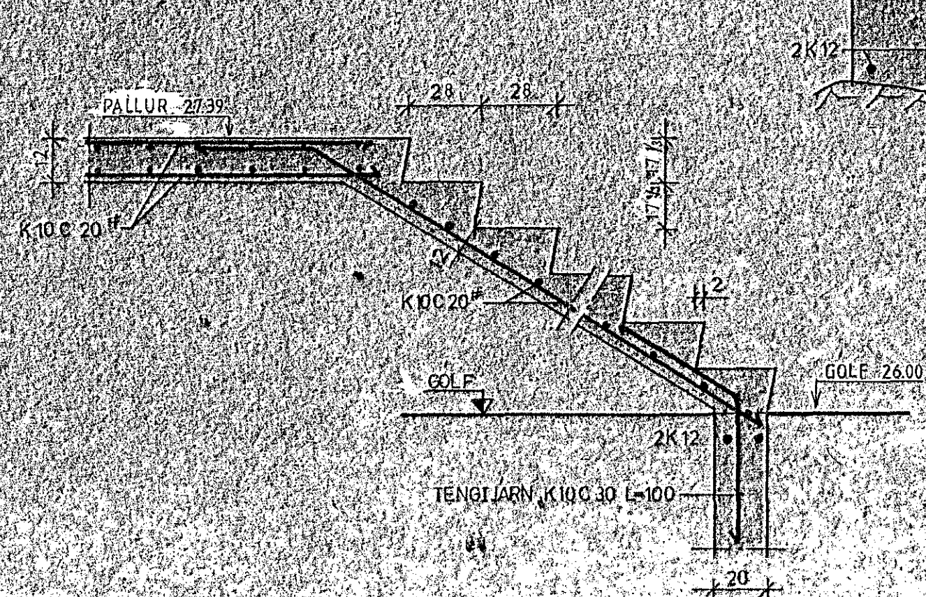
SNÍÐ G-G 1:20
