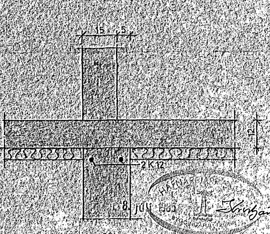
SNÍÐ D-D 1:10
