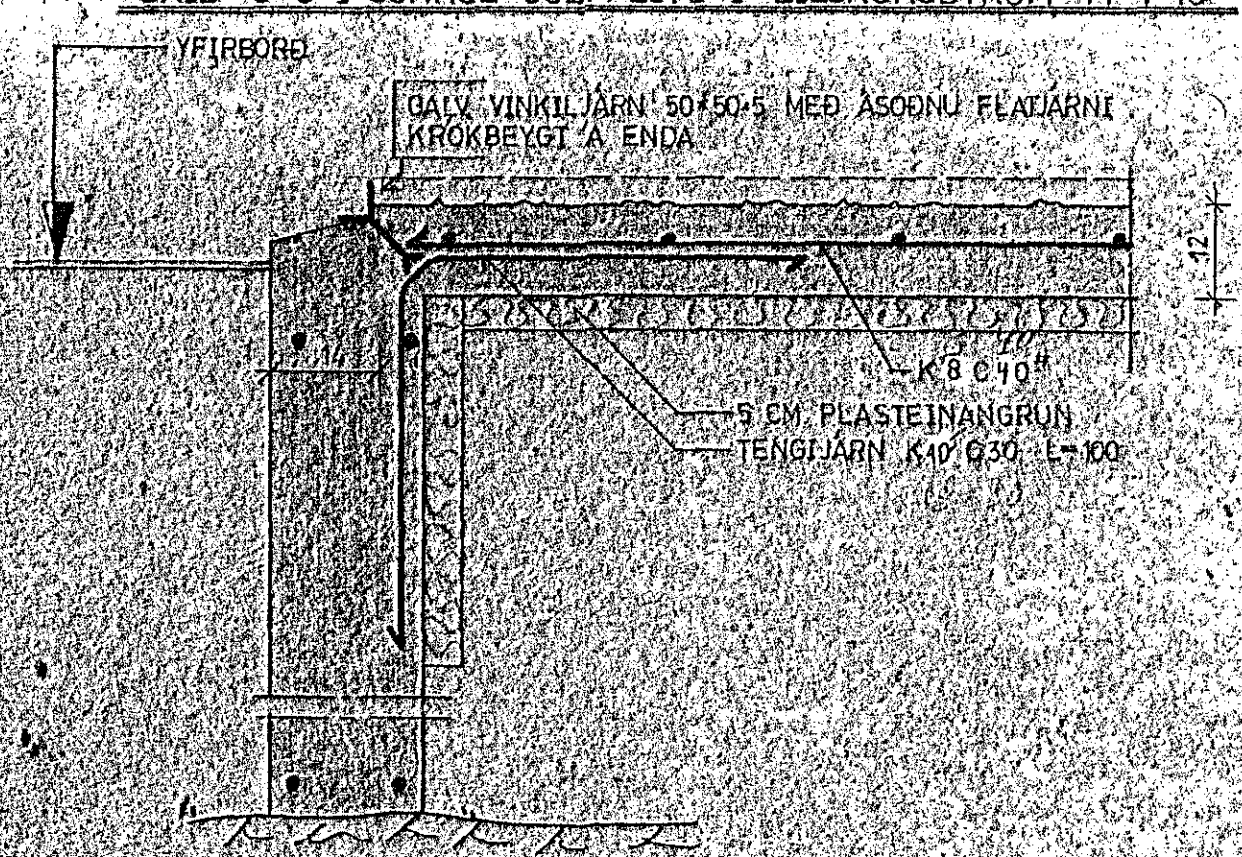
SNÍÐ G-G Í SÖKKUL GÖLFPLÖTU Í BÍLSKÚRSDYRUM M. 1:10
