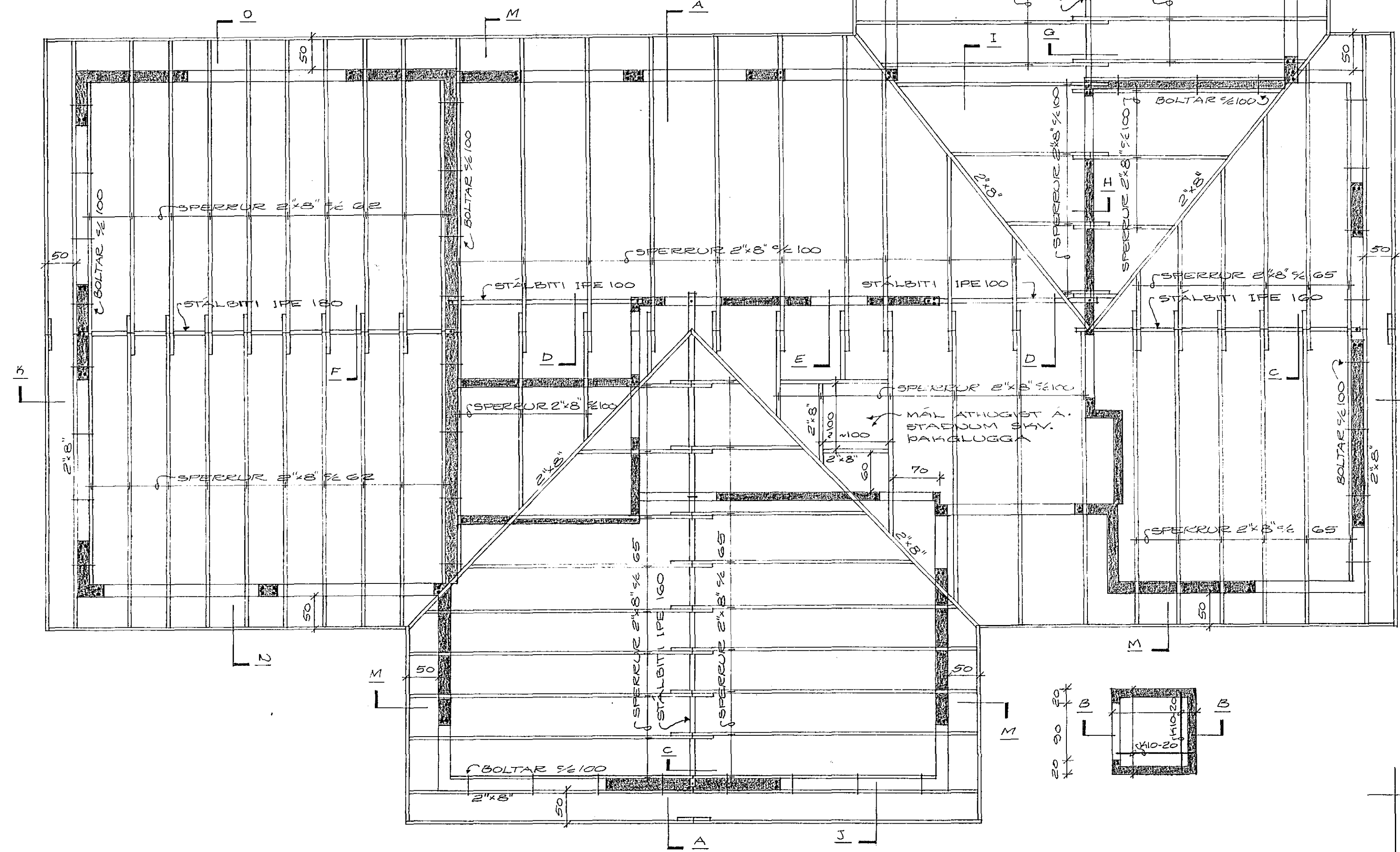
GRUNNMYND, M=1:50
