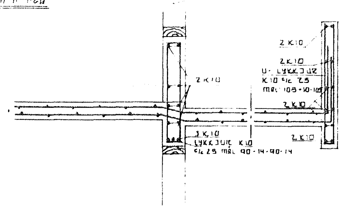
SNID A-A 1:20
