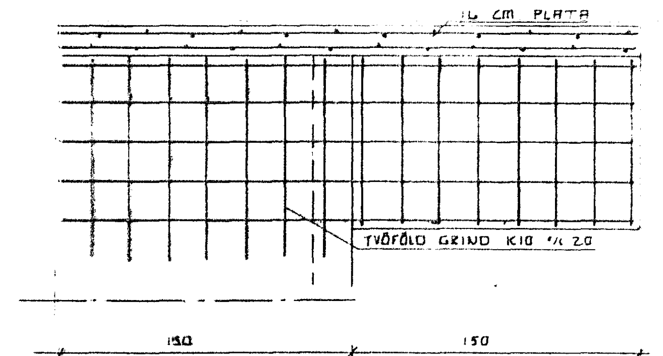
SNID B-B 1:20
