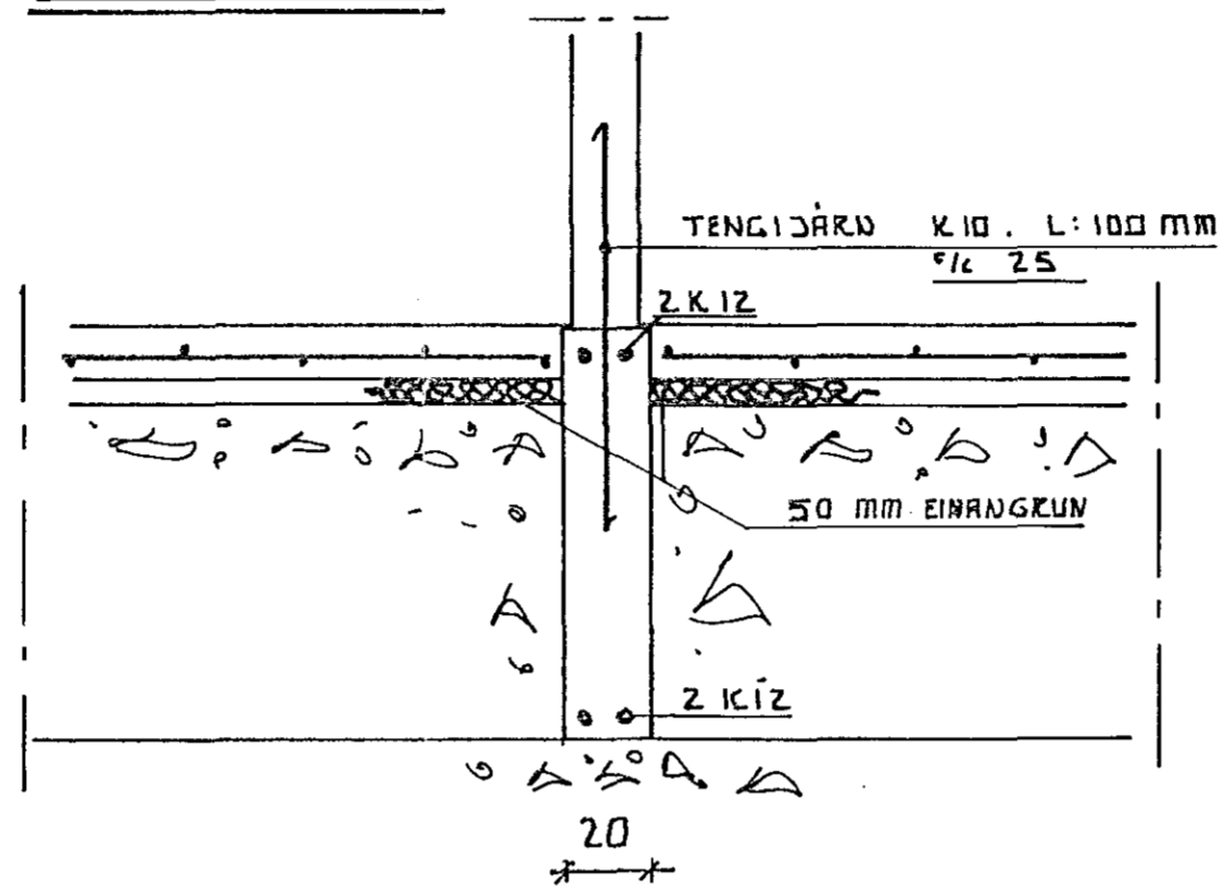
B-B 1:20
