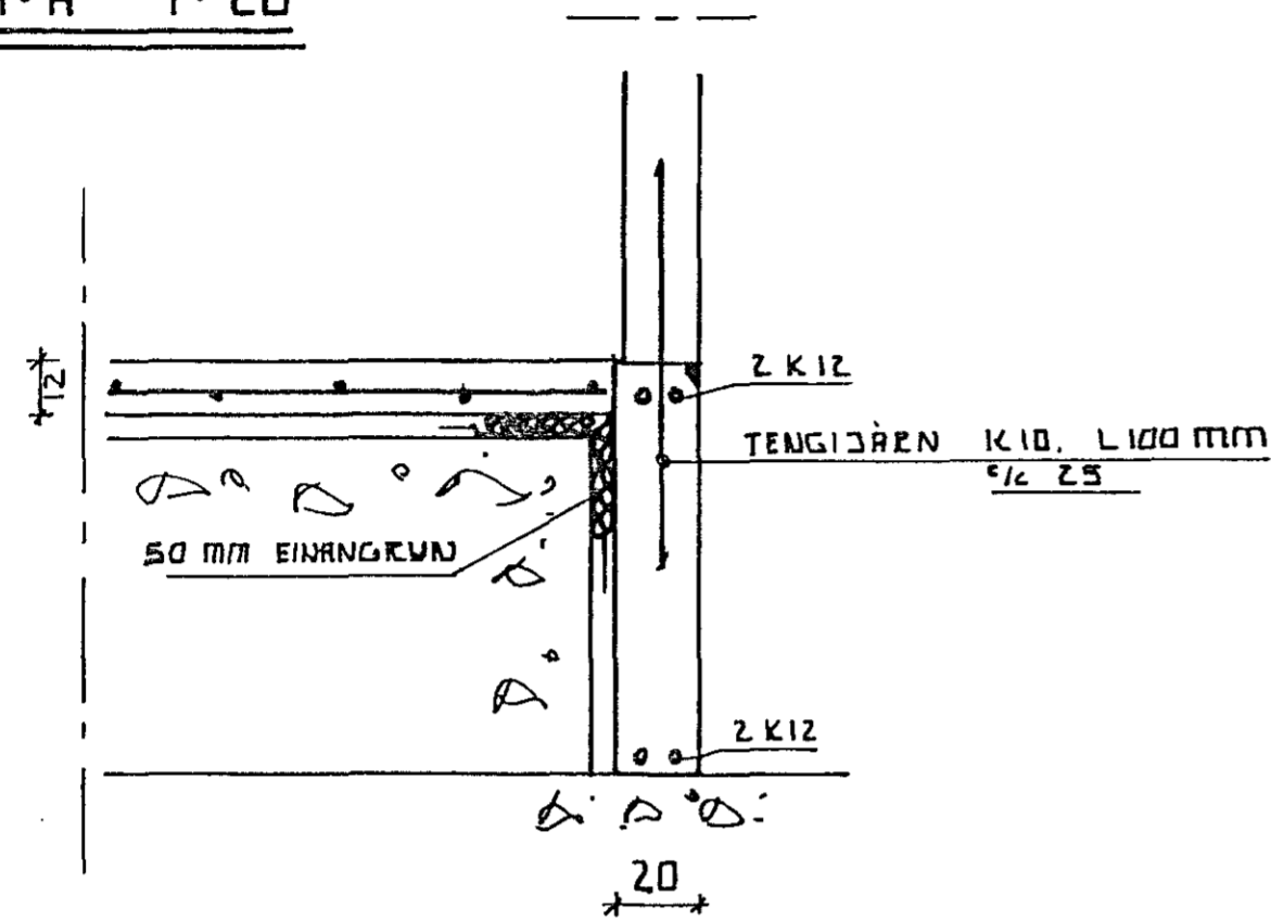
A-A 1:20
