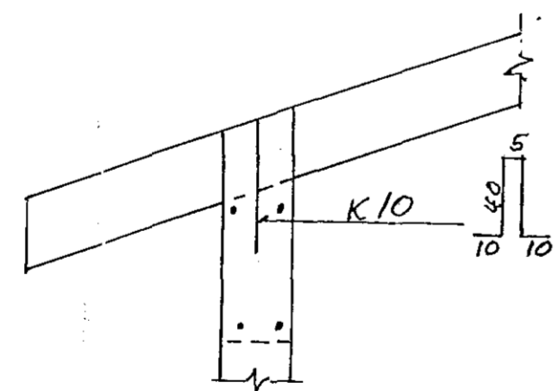
PAKFASTINGAR Í STEYPTA VEGGI 1:20
