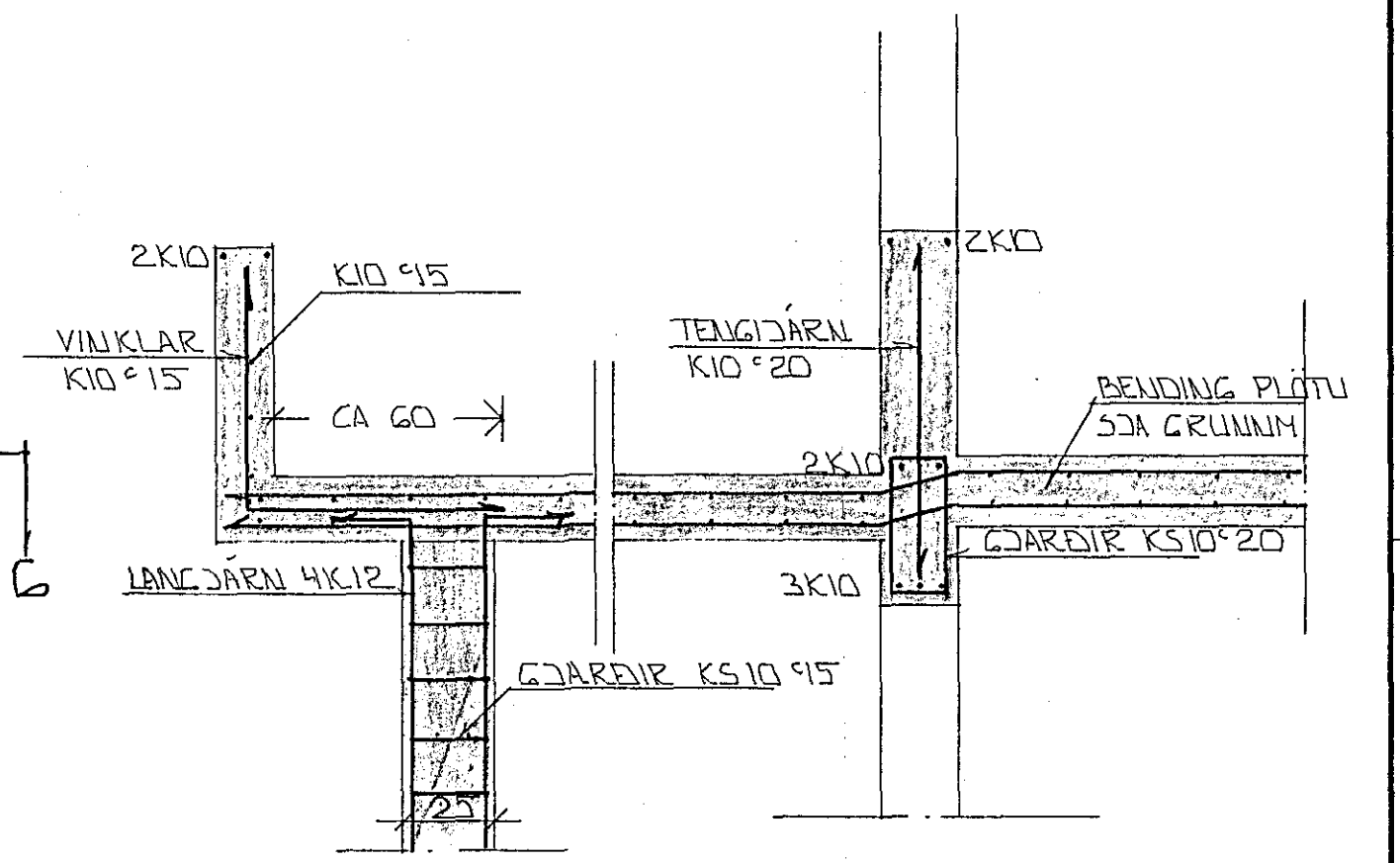
SNID G-G · 1:20
