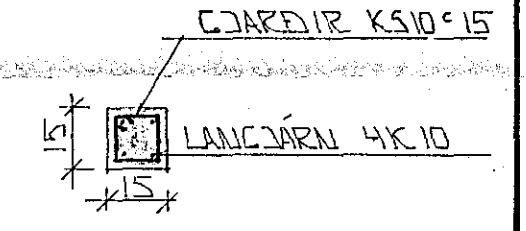
SÚLA S2 · 1:20
