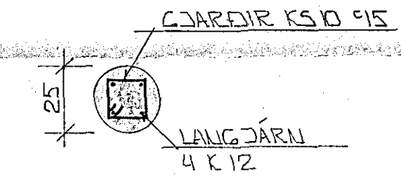
SÚLA S1 · 1:20
