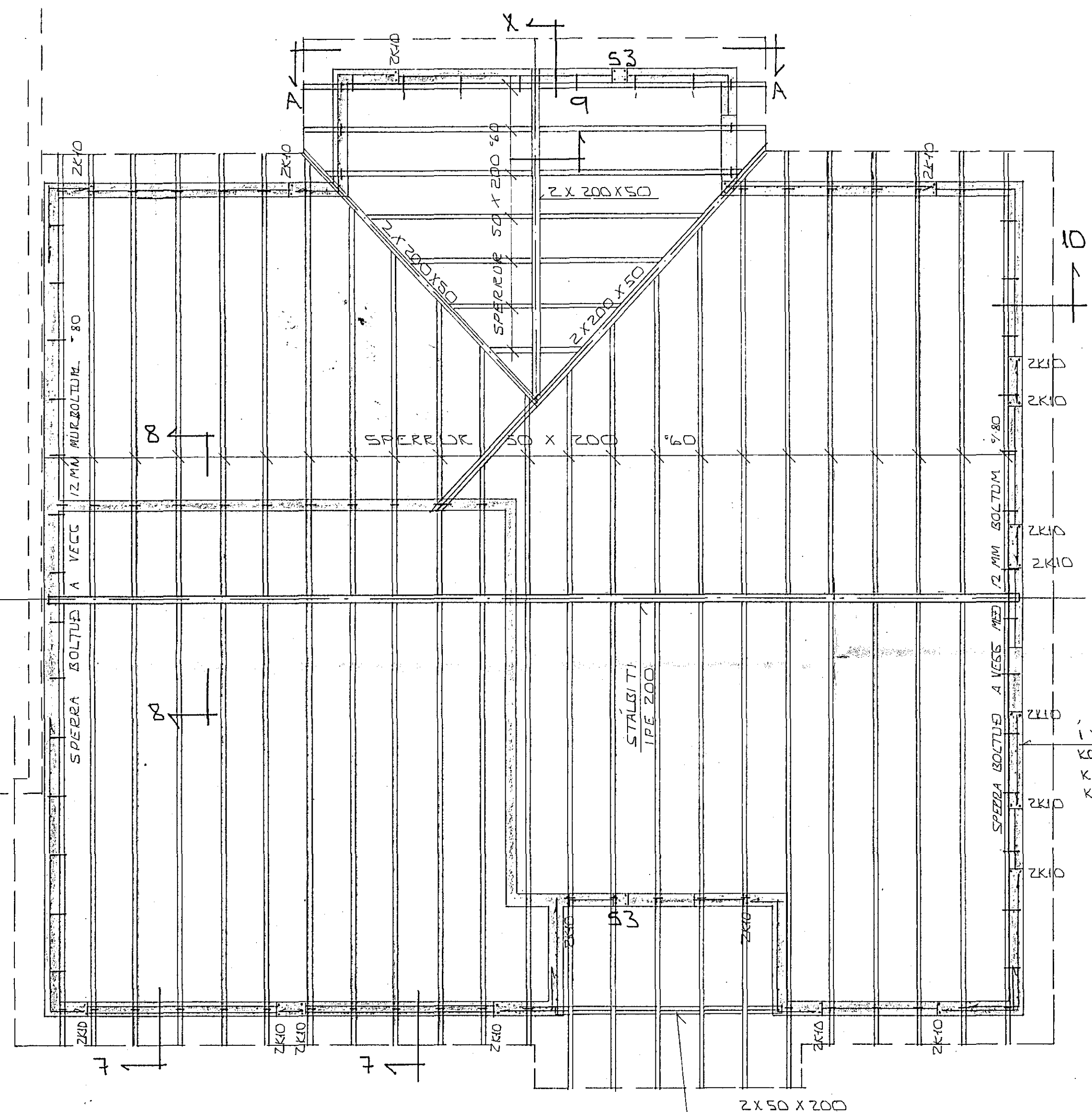
GRUNNMYND · 1 : 50
