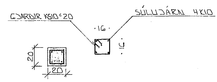
SÚLA S3 · 1 : 20
