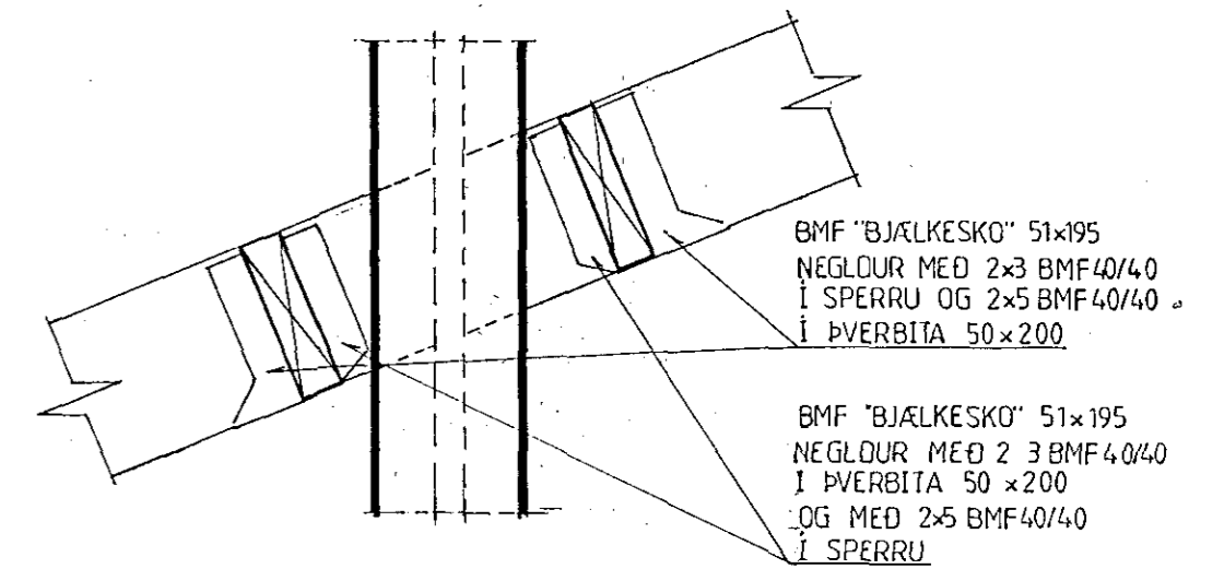
FRÁGANGUR Á SPERRUM VID SKORSTEIN M 1:10
