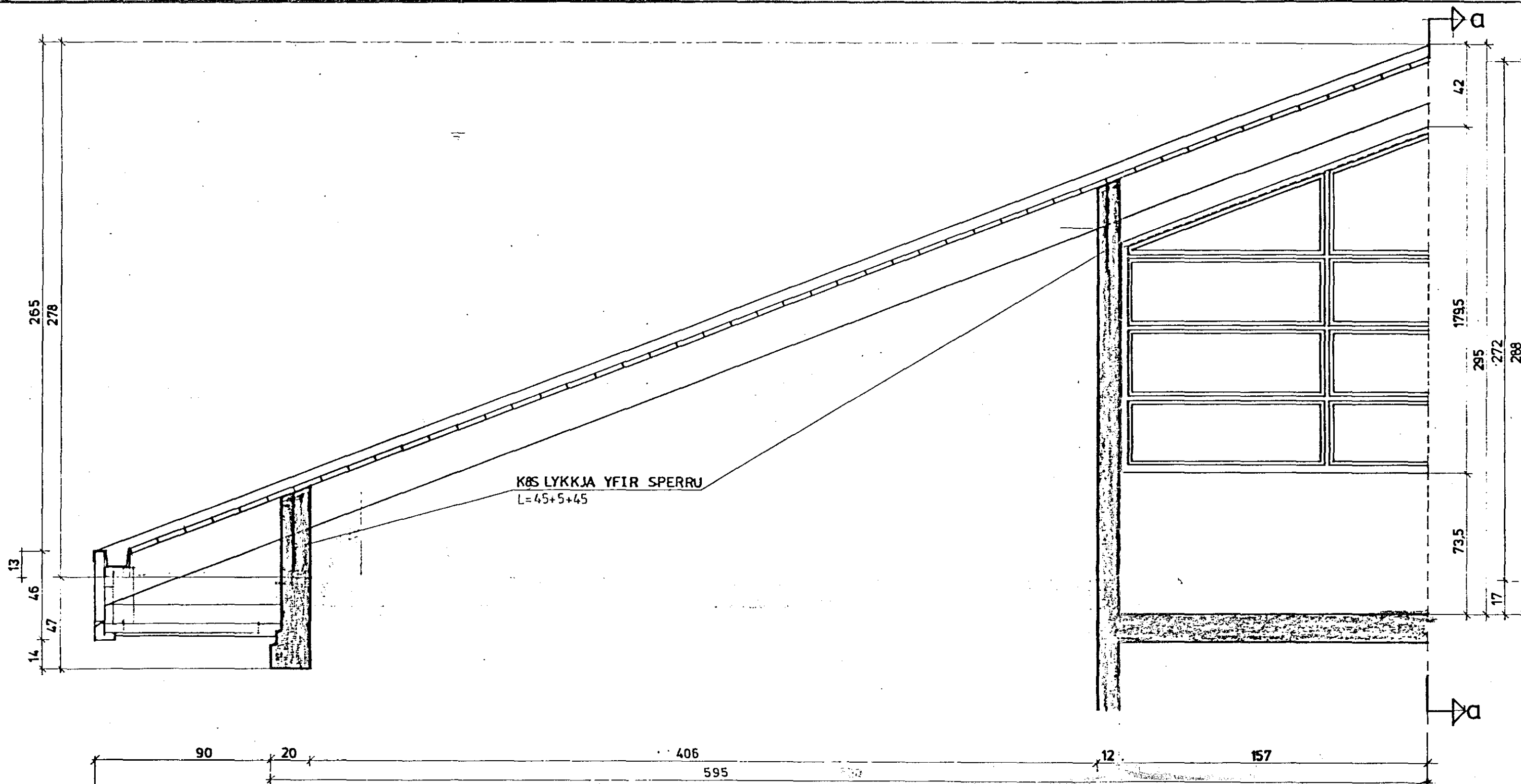
SNID A-A M 1:20
