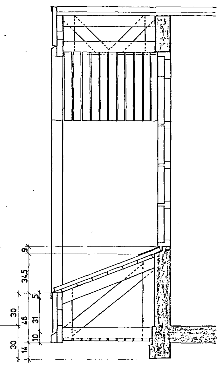
SNID a-a M 1:20
