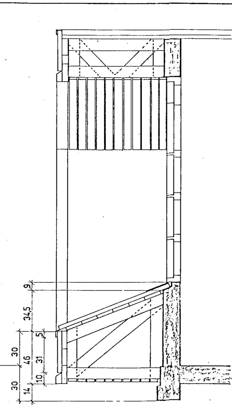
SNID a-a M 1:20
