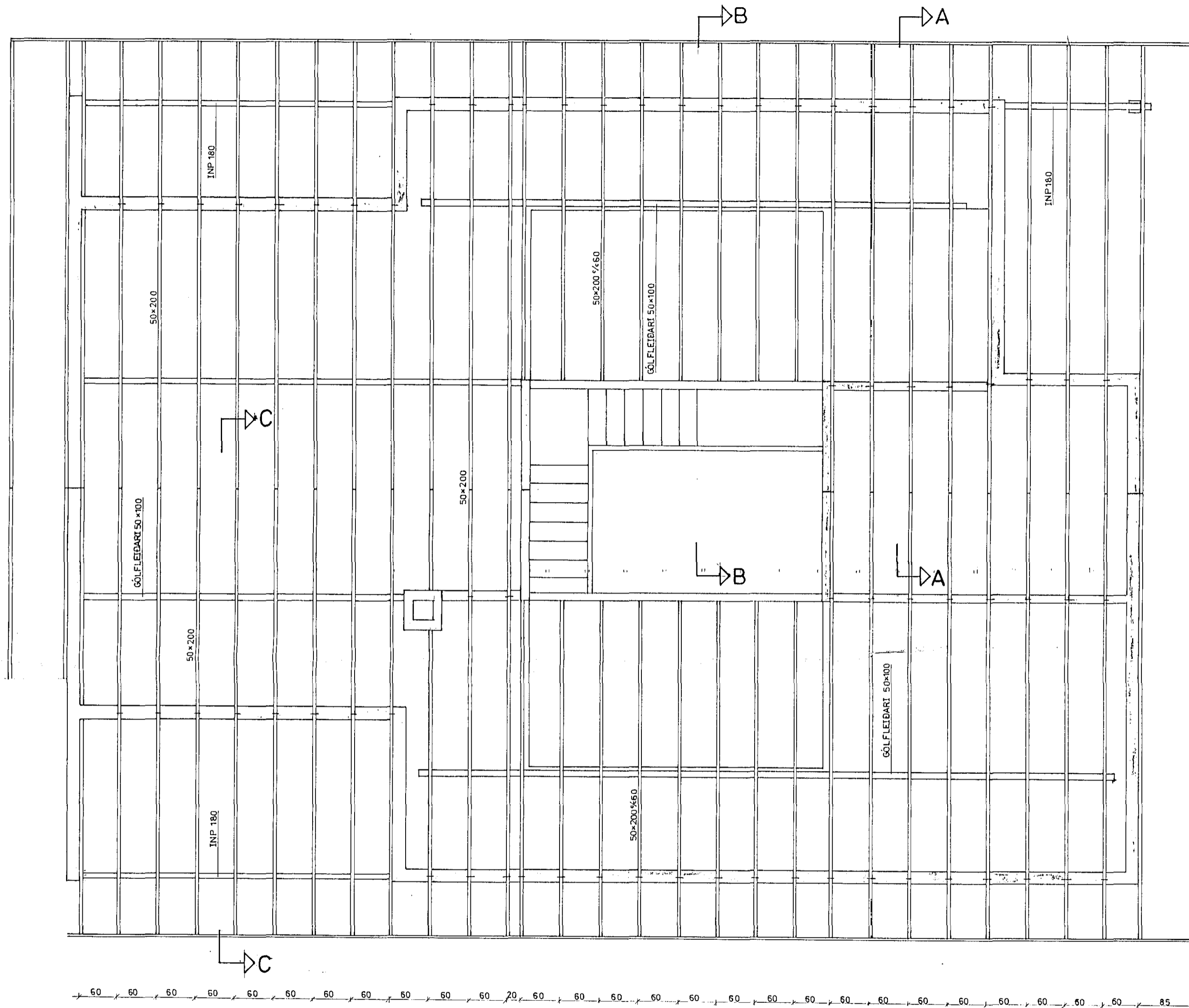
SPERRUPLAN M 1:50
