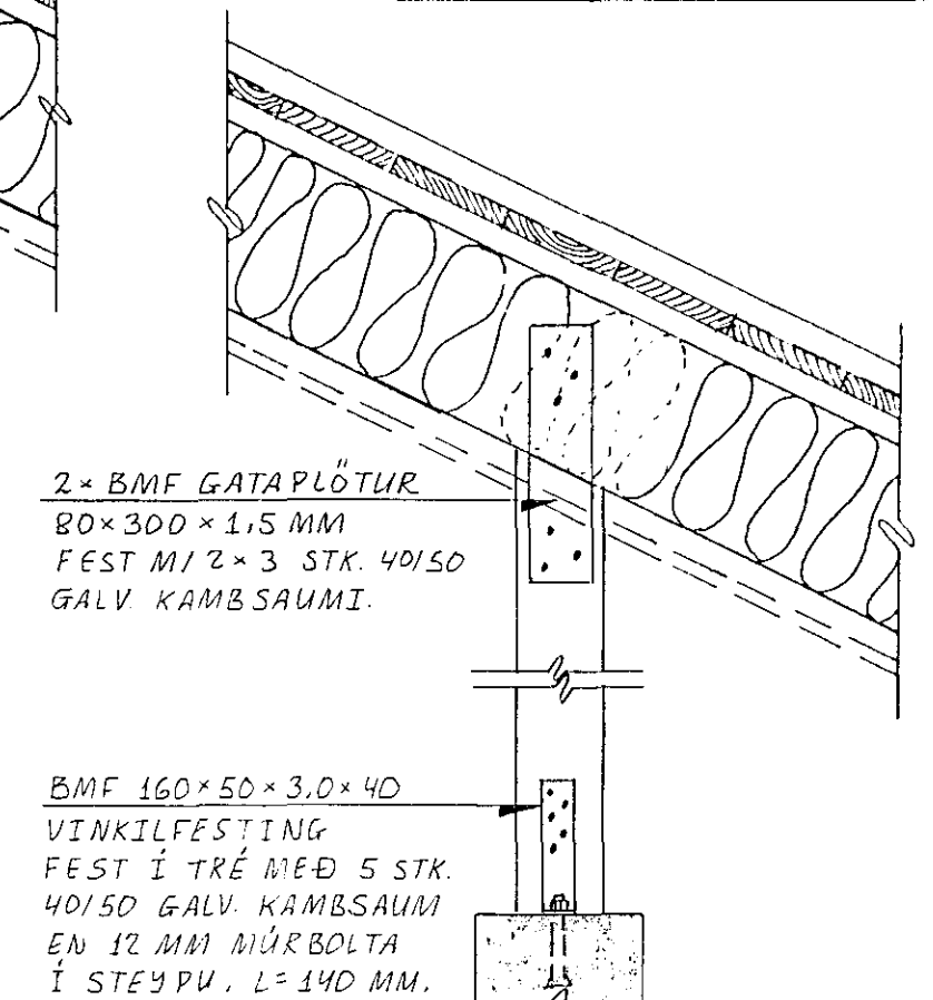
SNID F 12 -F 12 . 1:10
