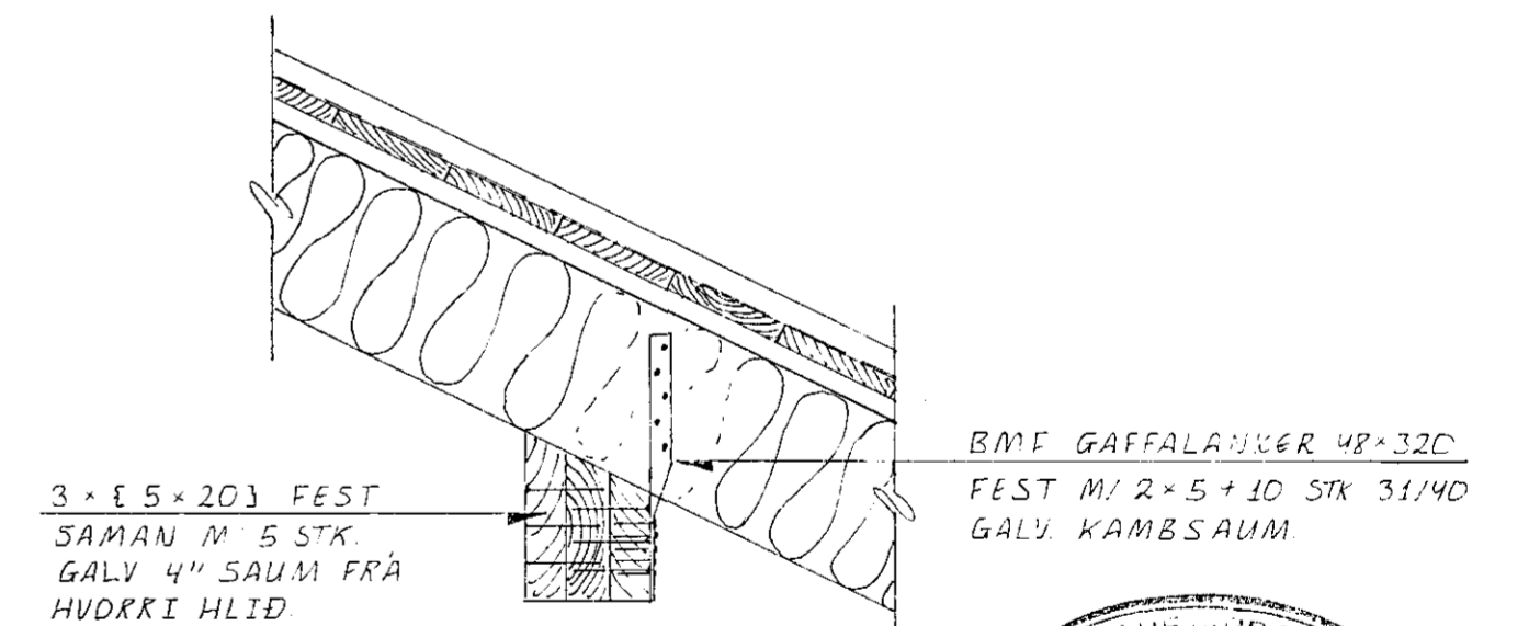
SNID G 12 -G 12 . 1:10
