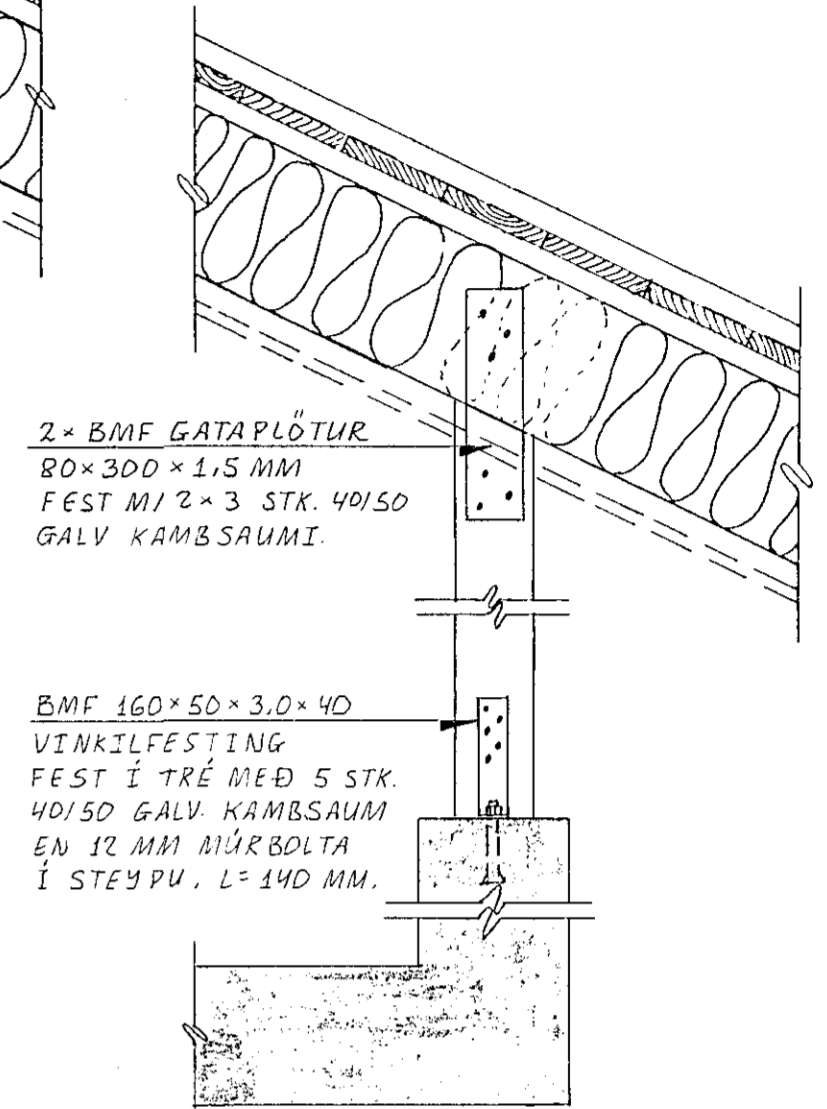
SNID F 12 -F 12 . 1:10
