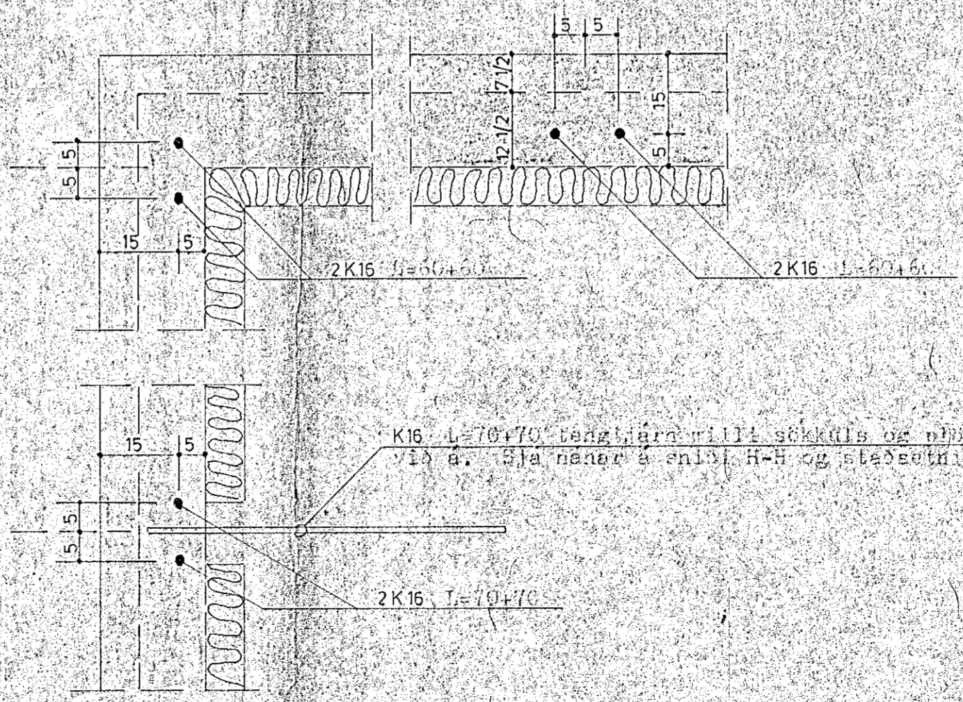
TENGJARN MILLE BOKKULS OG LITJGAR, M=1:10. sjá staðsetningu tengjarnanna á grunnmynd (tekn. nr. 101).
