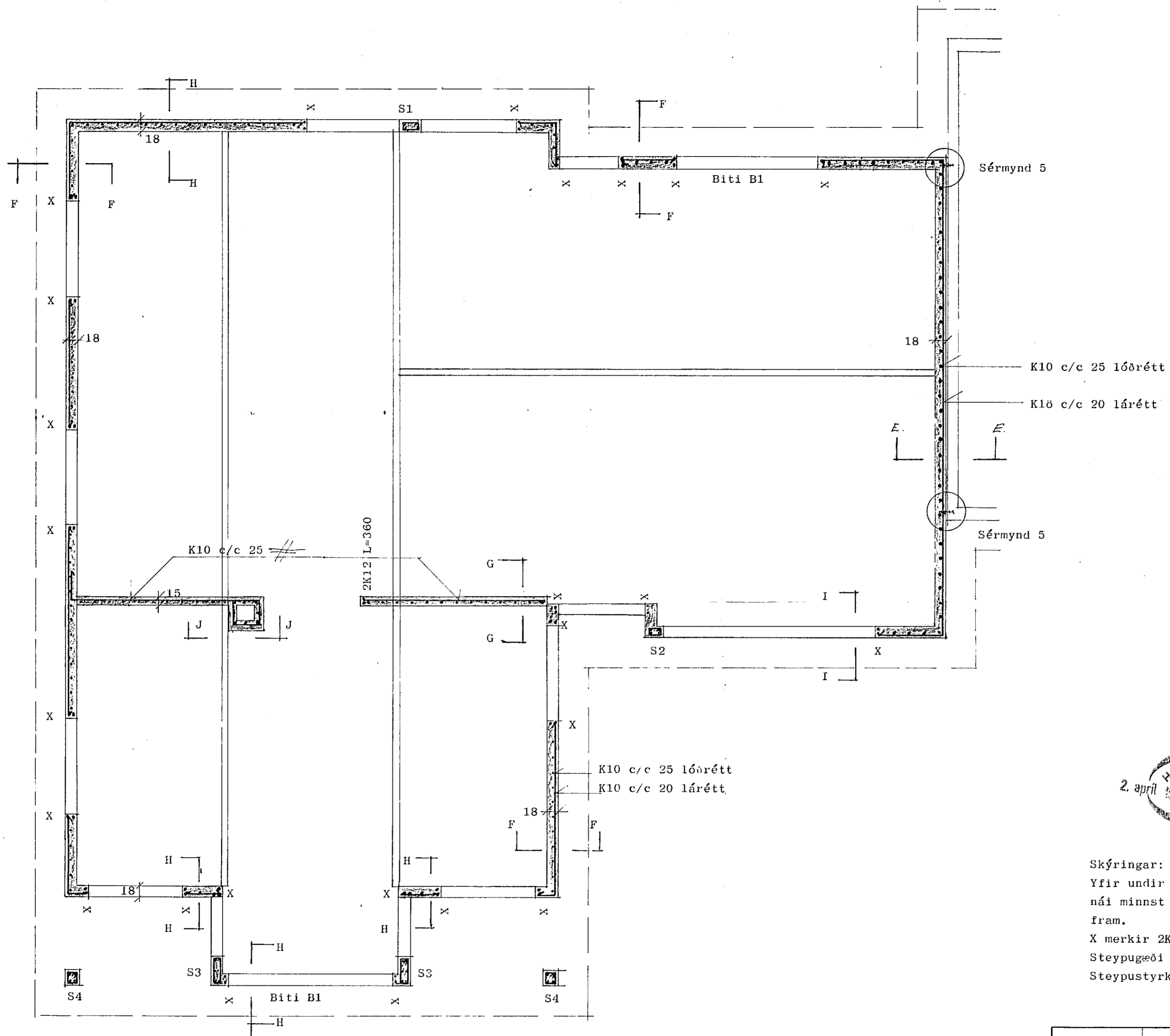
Grunnmynd 1:50
