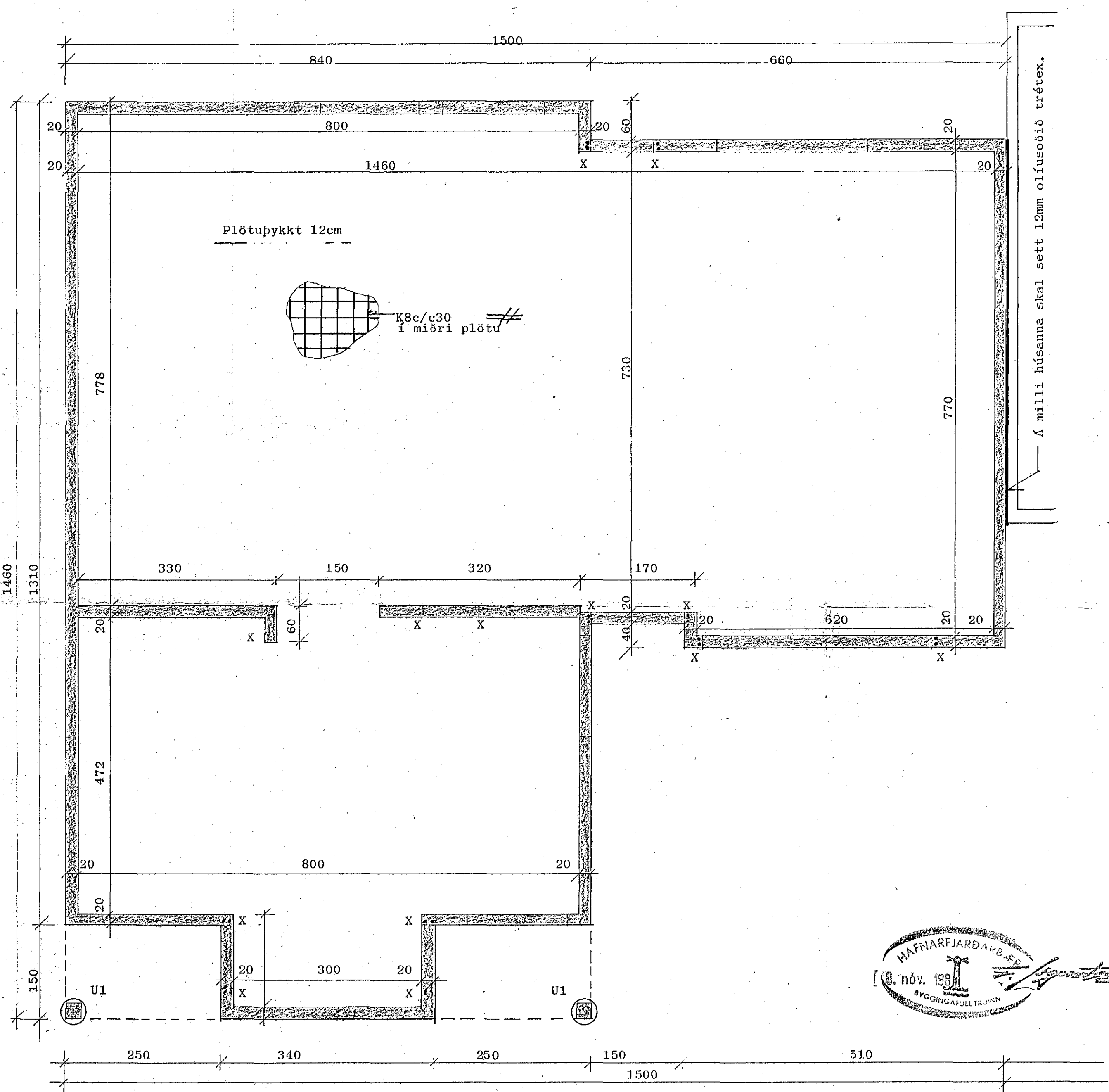
Grunnmynd 1:50
