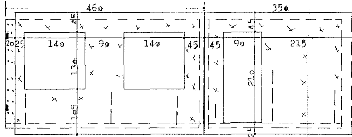
Rauf fyrir hita og neysluvatn | Rauf fyrir hitalagnir
