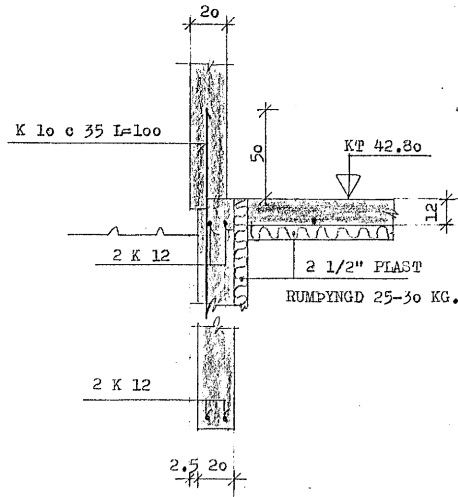
SNID A-A 1:20
