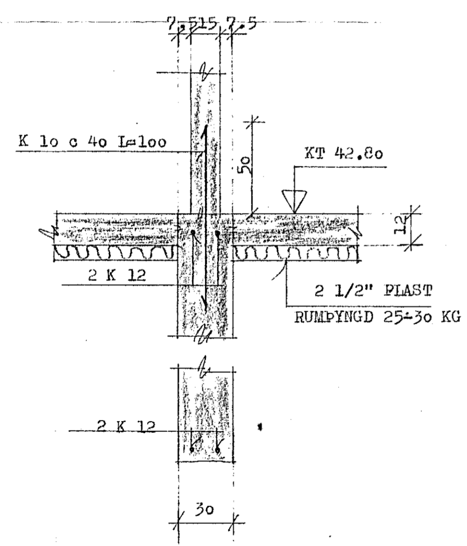
SNID D-D 1:20
