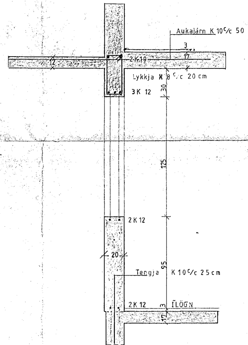
Sníð A-A 1:20
