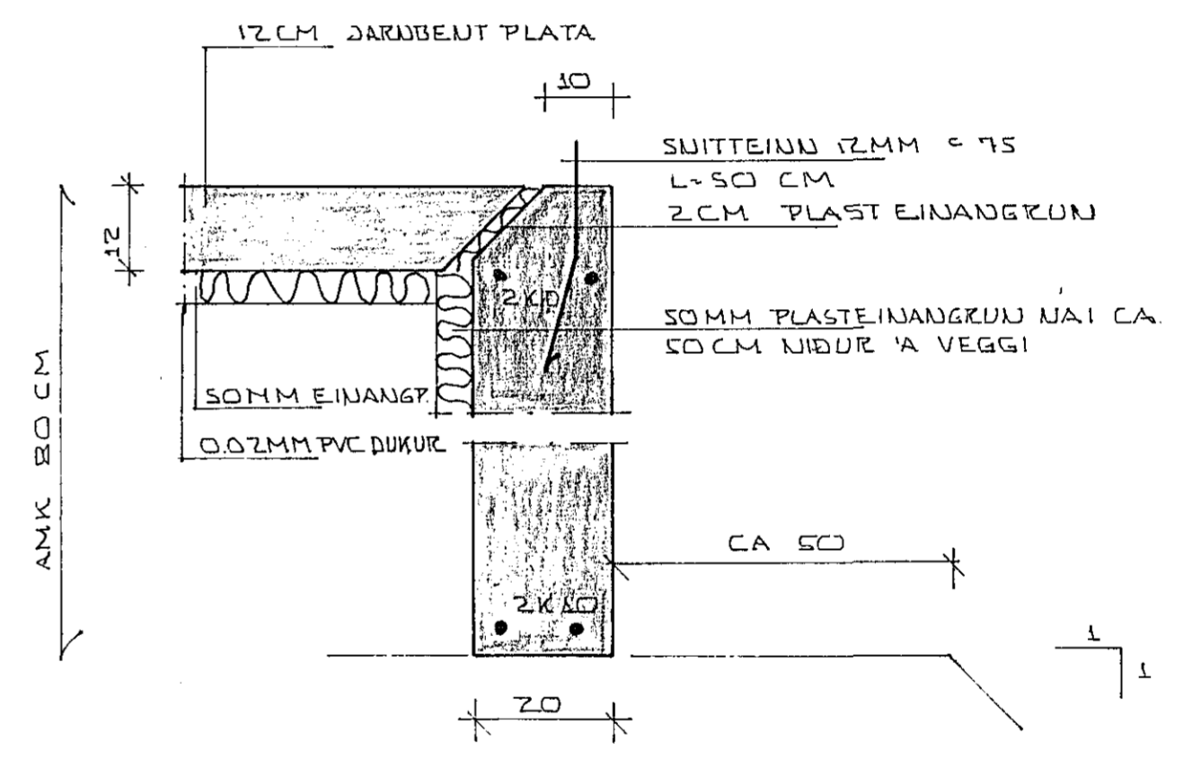
SNID Í ÚTVEGG 1:10
