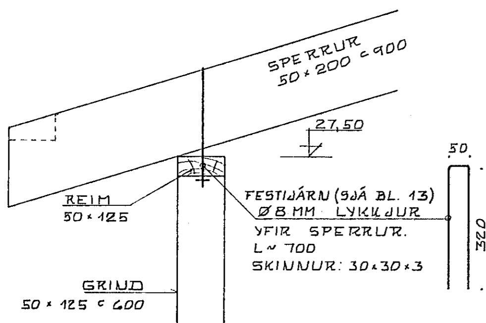
SÉRMYND A 1:10
