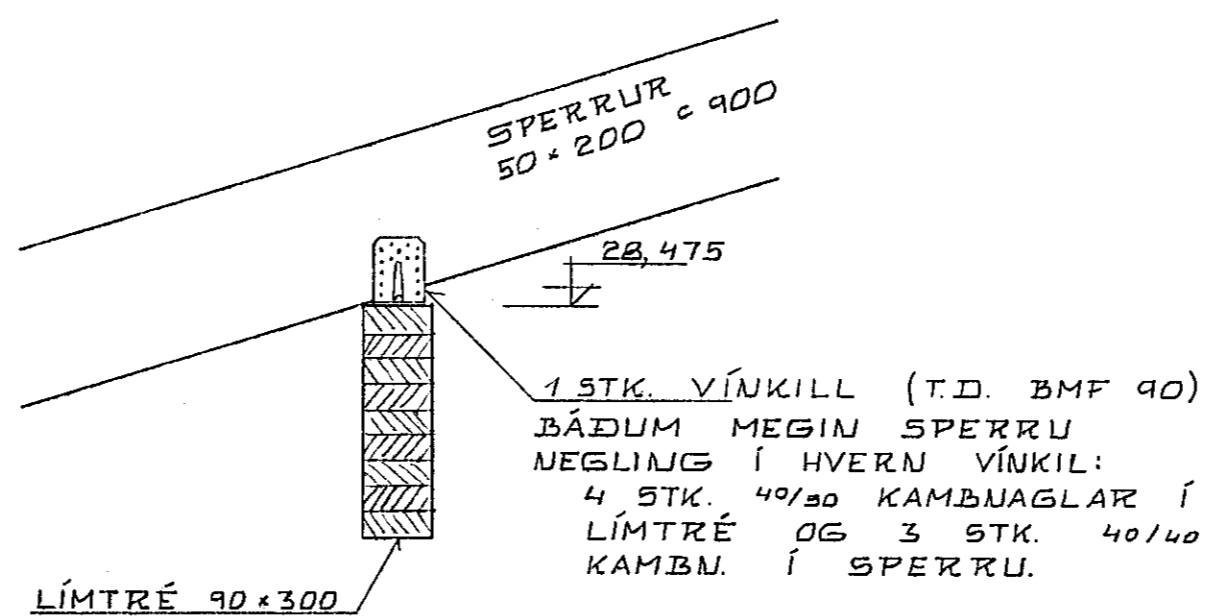
SÉRMYND B 1:10
