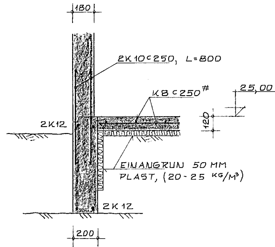
SNID 1-1 1:20
