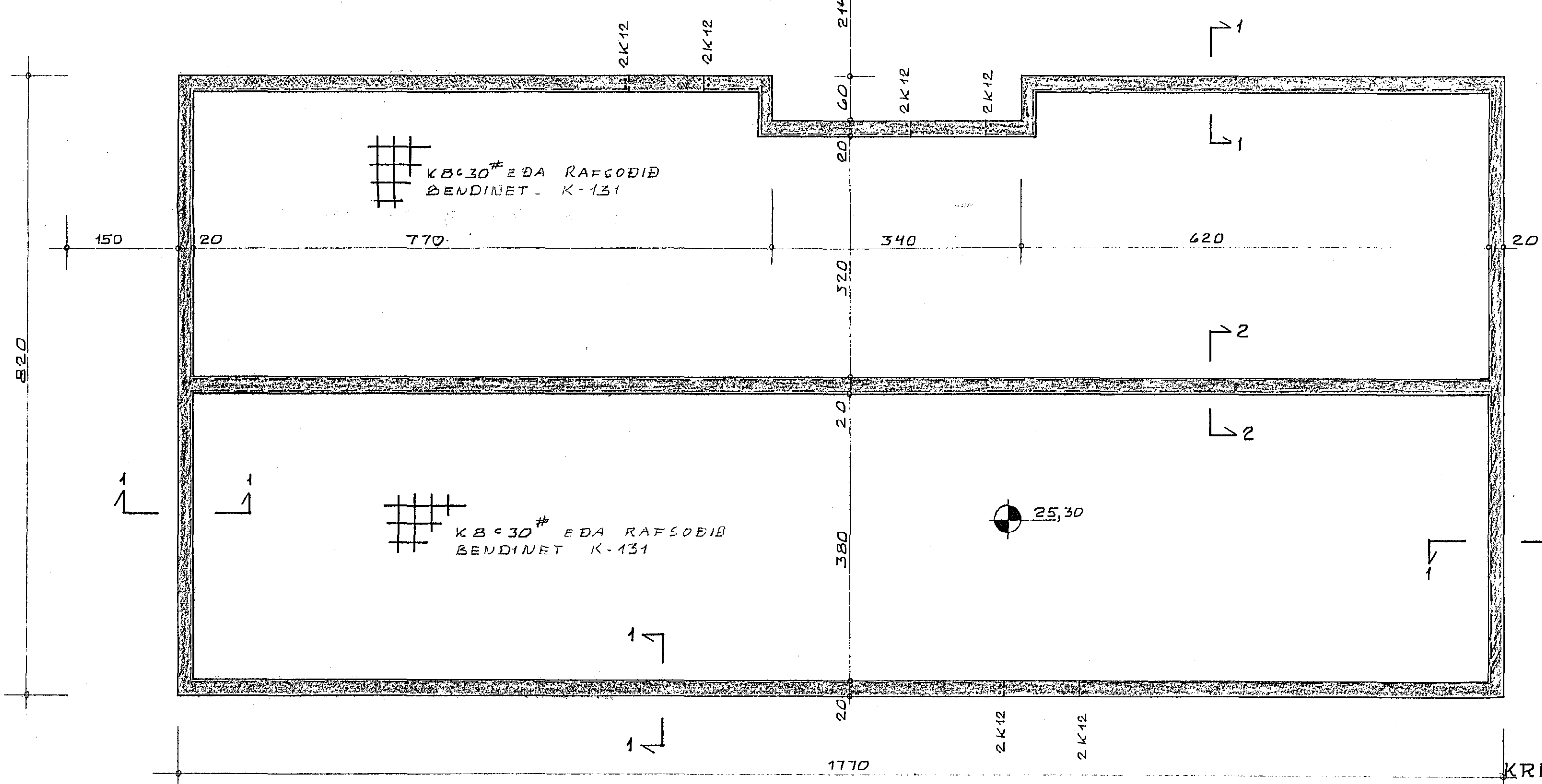
GRUNNMYND 1:50
