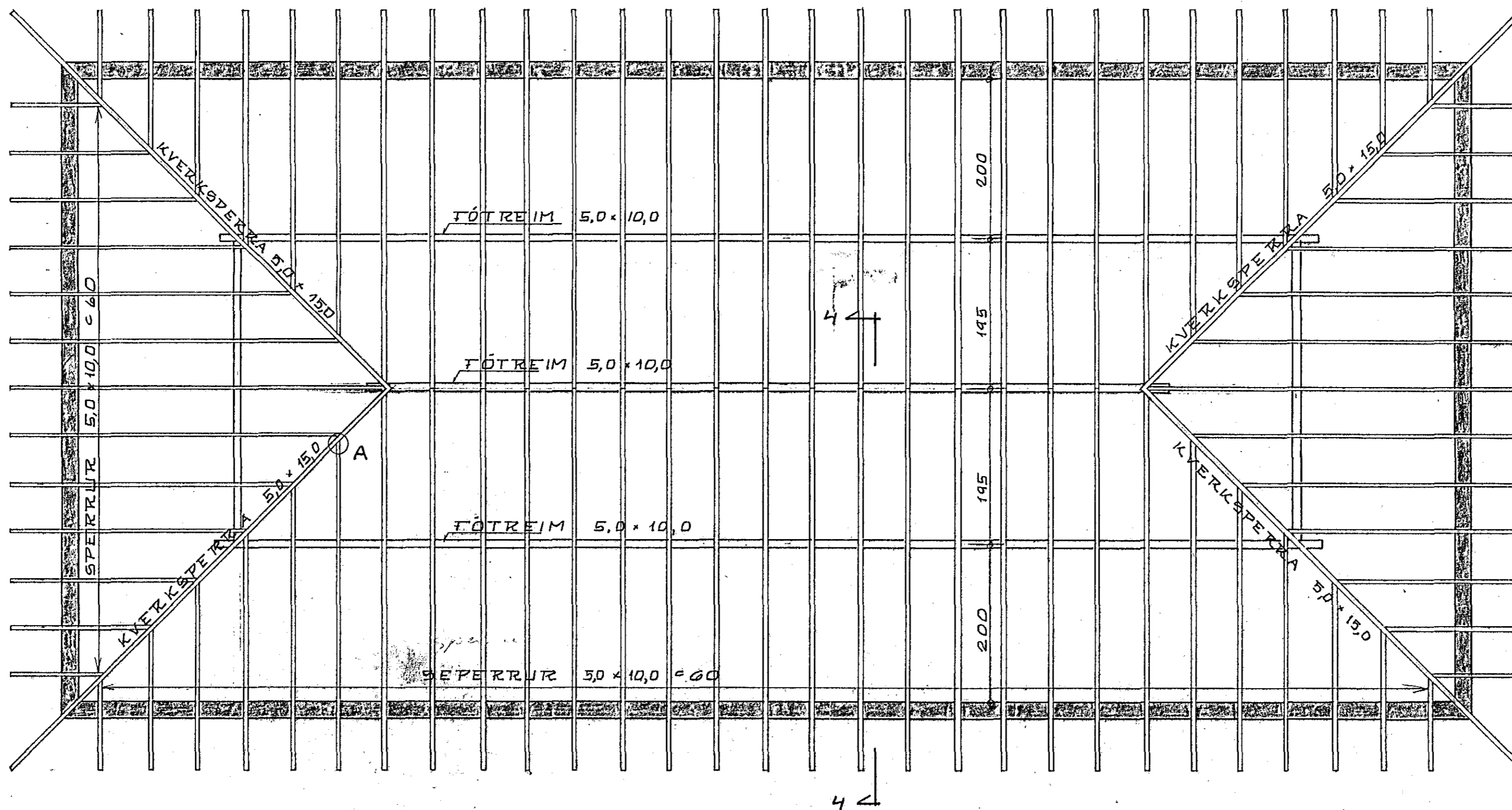
GRUNNMYND 1:50
