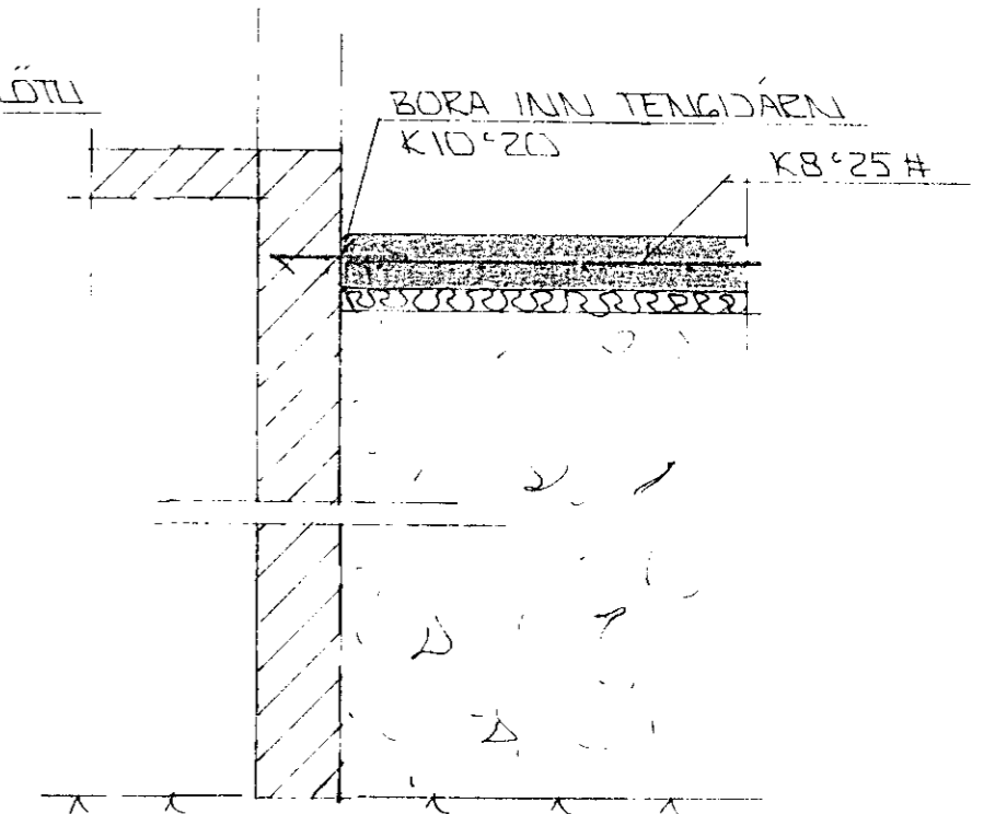
SNID 2 1:20
