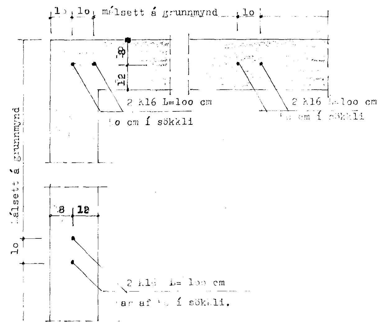
TENGIÁRNA UPP ÚP SÖKKLI M 1:10
