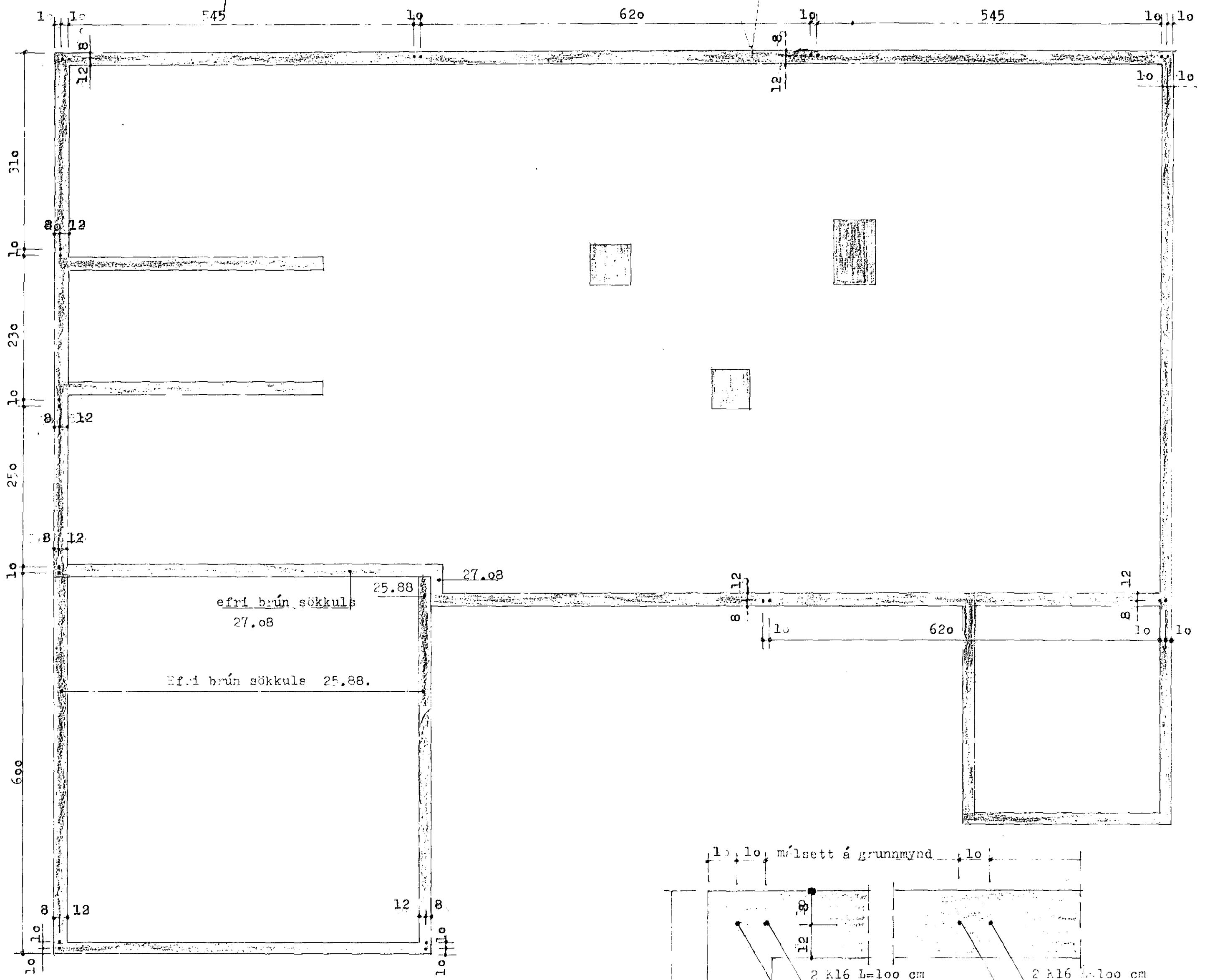
STOÐSETNING TENGIÁRNA M 1:20
