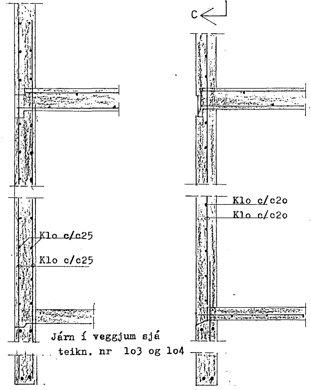
SNÍÐ C-C M 1:20
