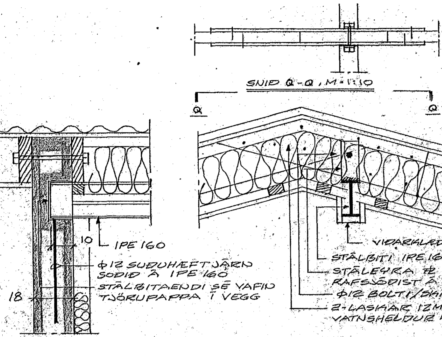
STÁLBITAFESTING Í ÚTVEGG, M=1:10
