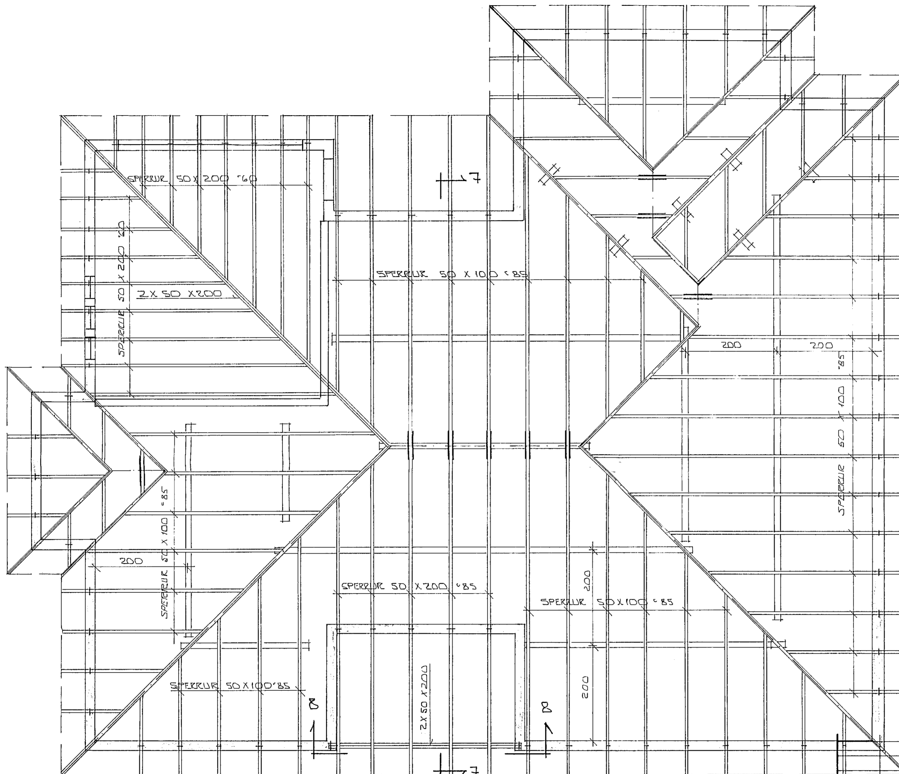
GRUNNMYND 1:50
