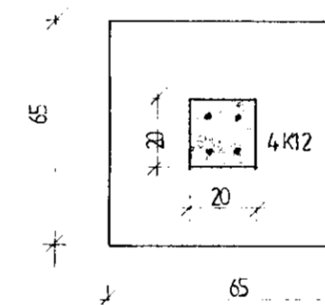
Súla S1 1:20
