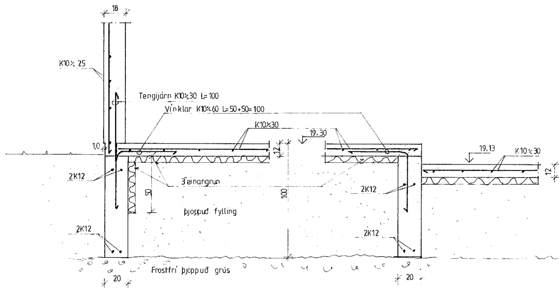
Snid B - B 1:20
