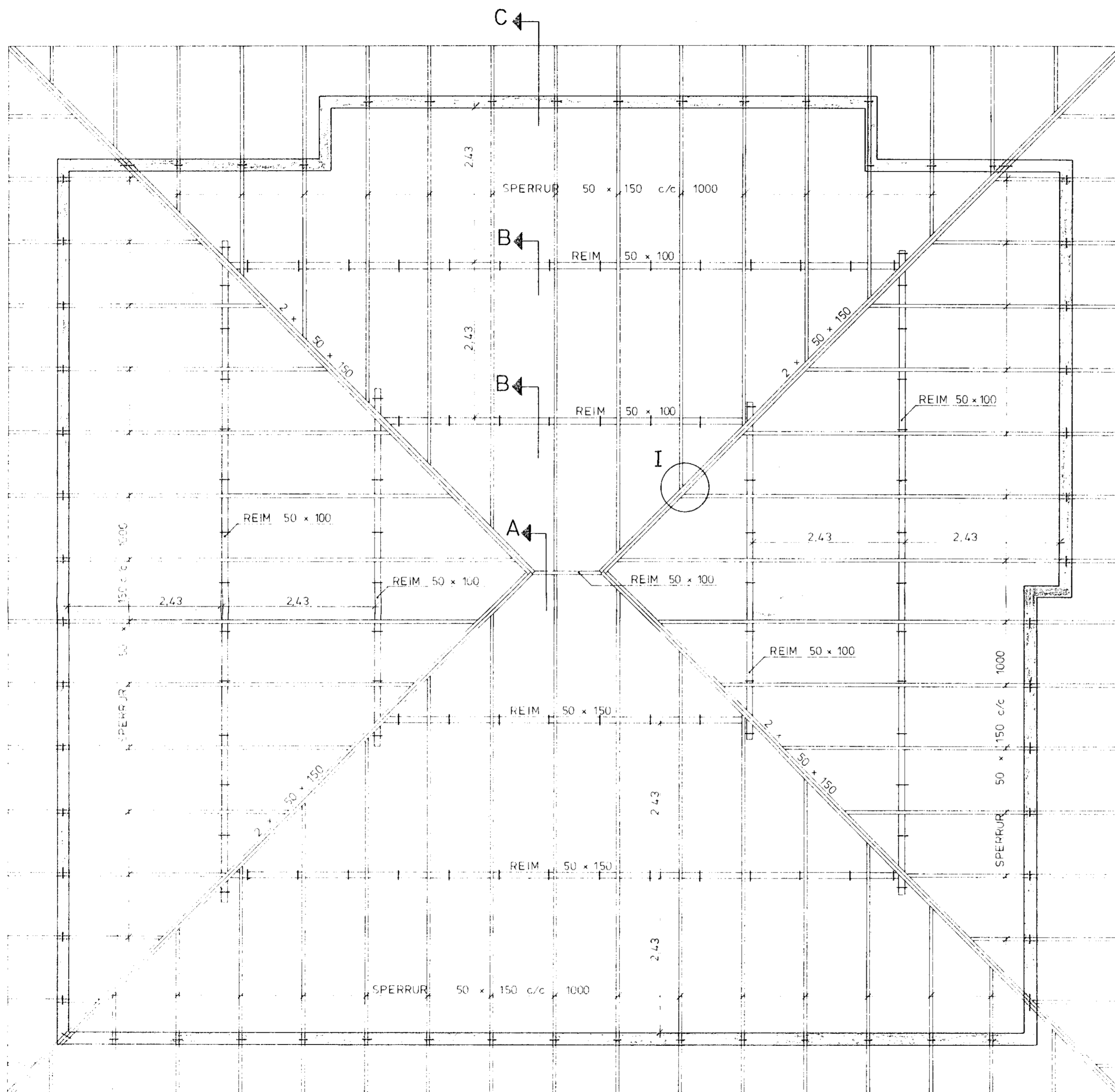
GRUNNMYND 1:50
