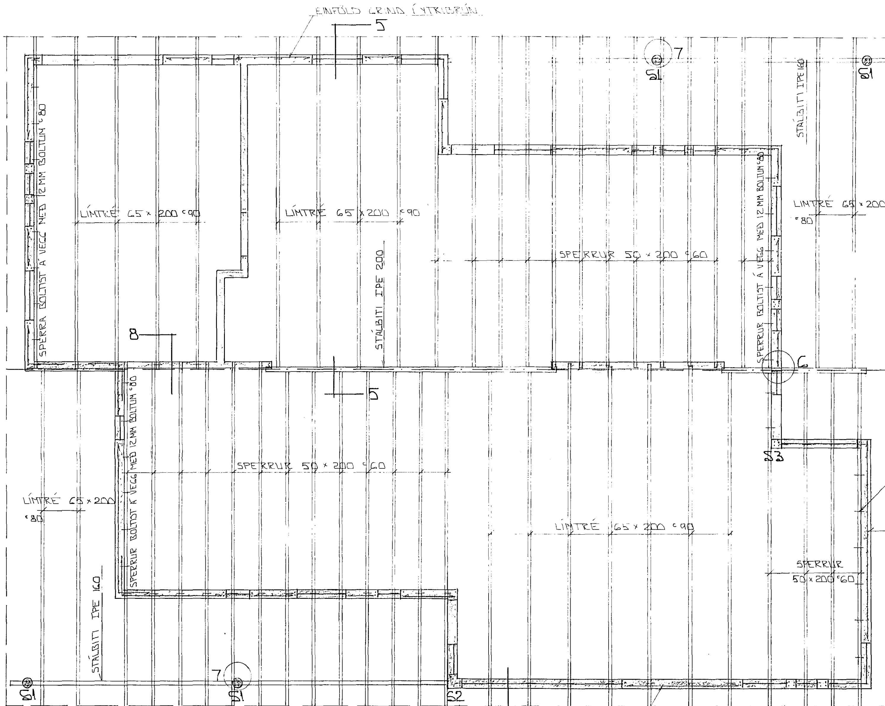
GRUNNMYND 1:50
