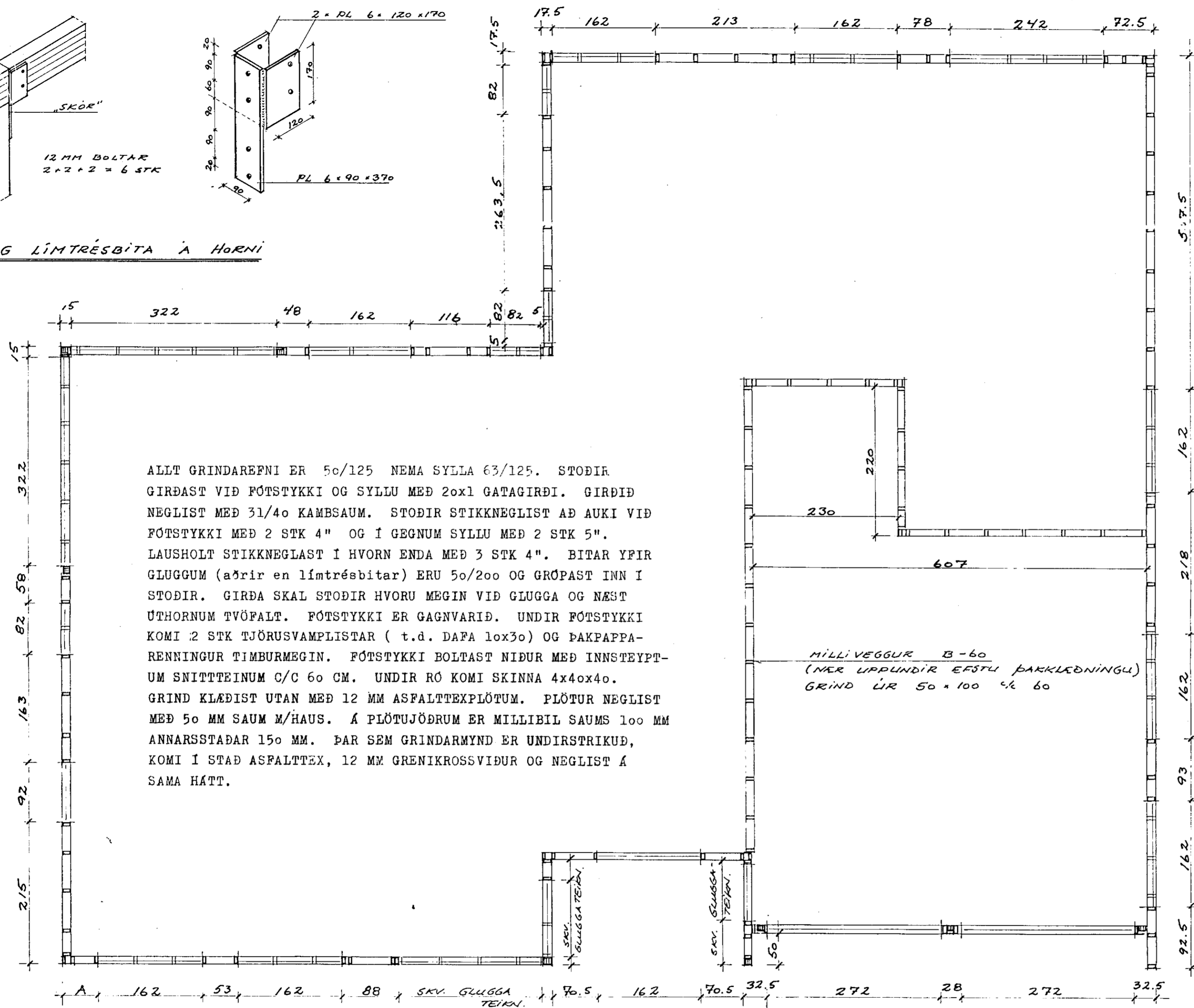
GRUNNMYND 1:50
