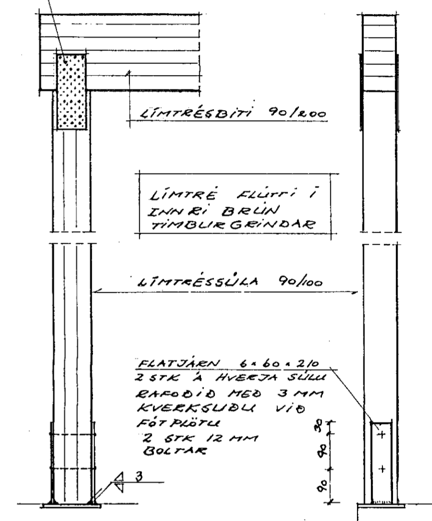
FESTING LÍMTRÉS 1:10
