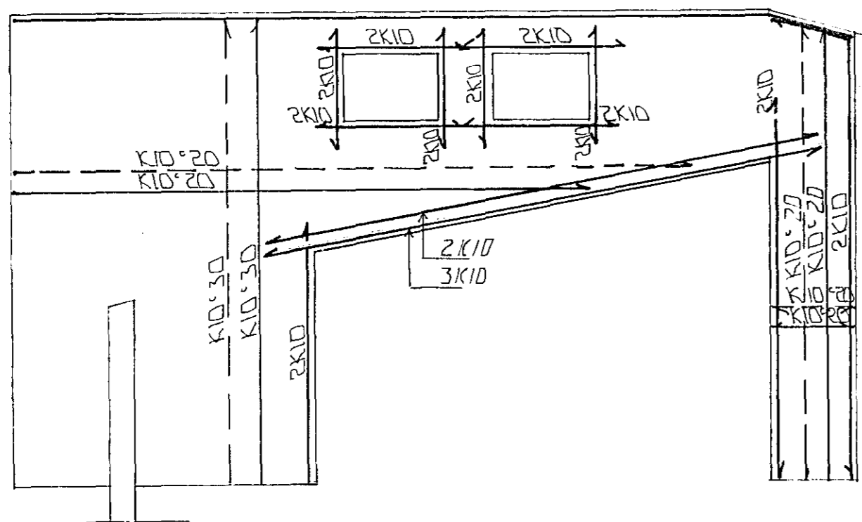
ÁSYND A-A · 1:50
