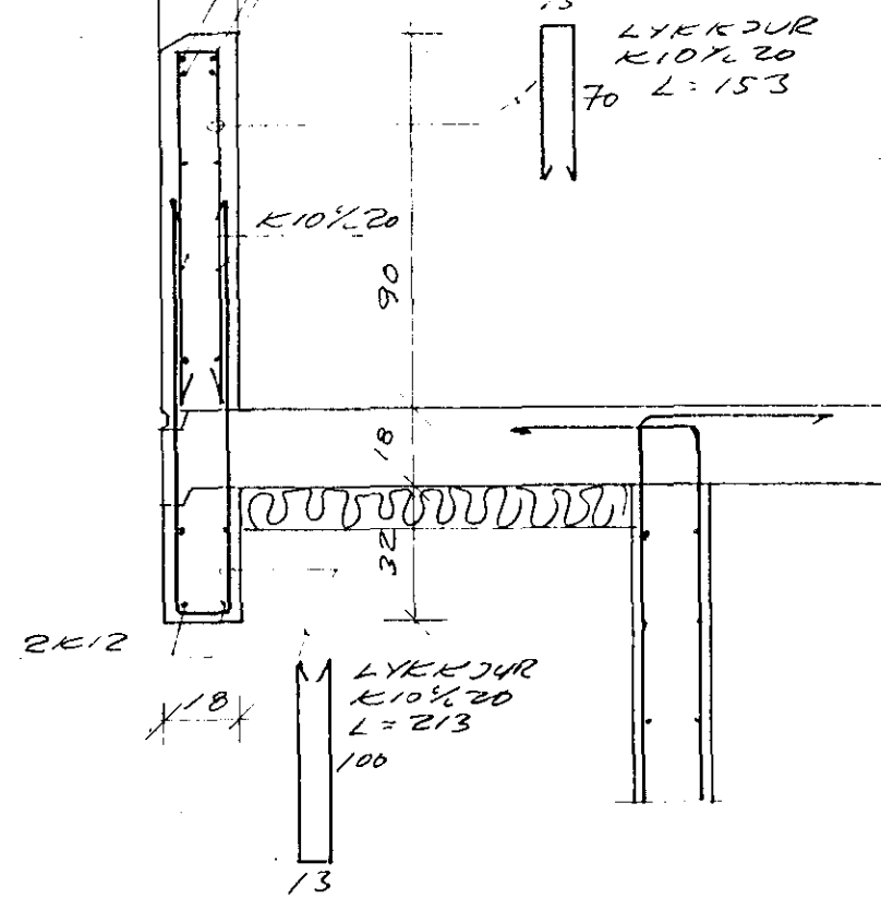
SNID U-U 1:20
