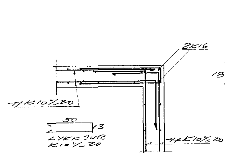
SNID P-P 1:20
