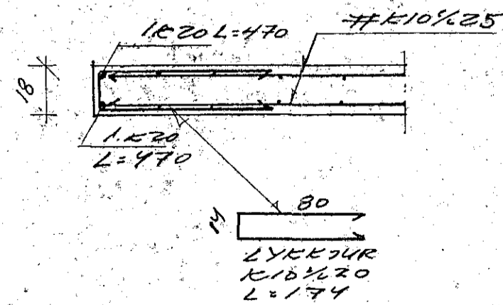
DEILI B2 1:20
