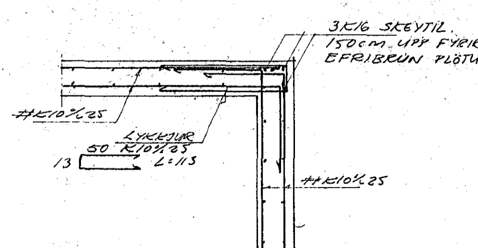
DEILI D2 1:20
