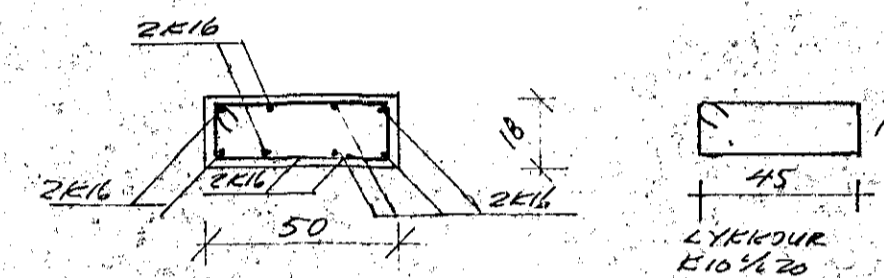
SÚLA S2A 1:20
