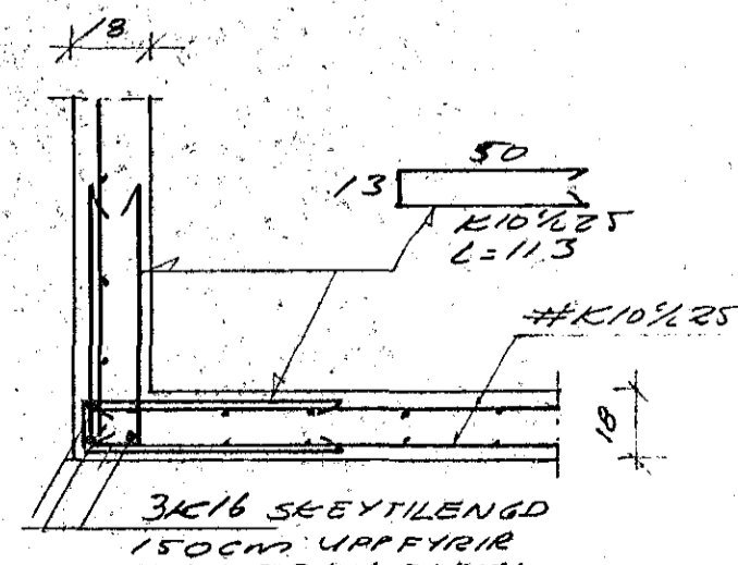
DEILI C2 1:20
