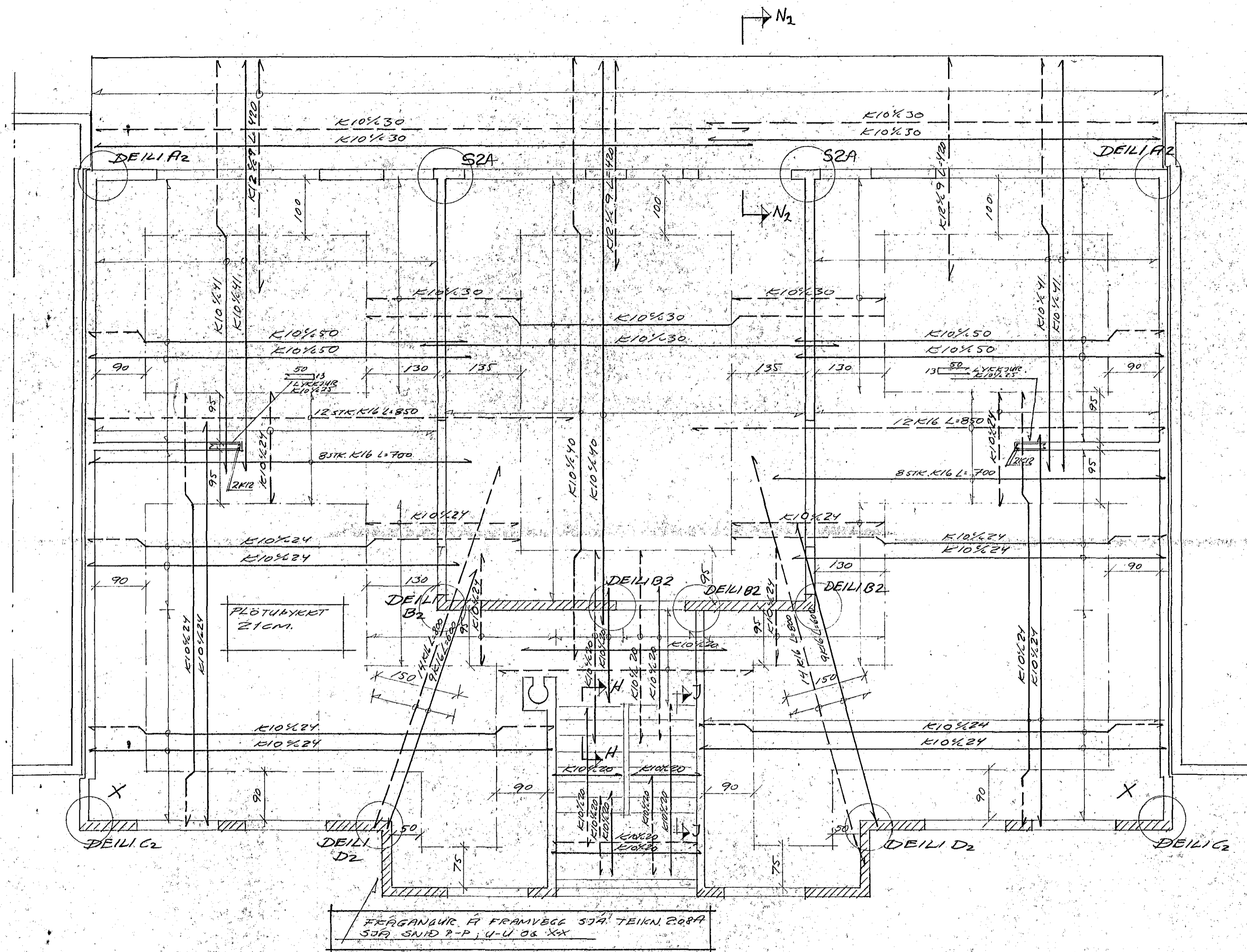
DEILI A2 1:20
