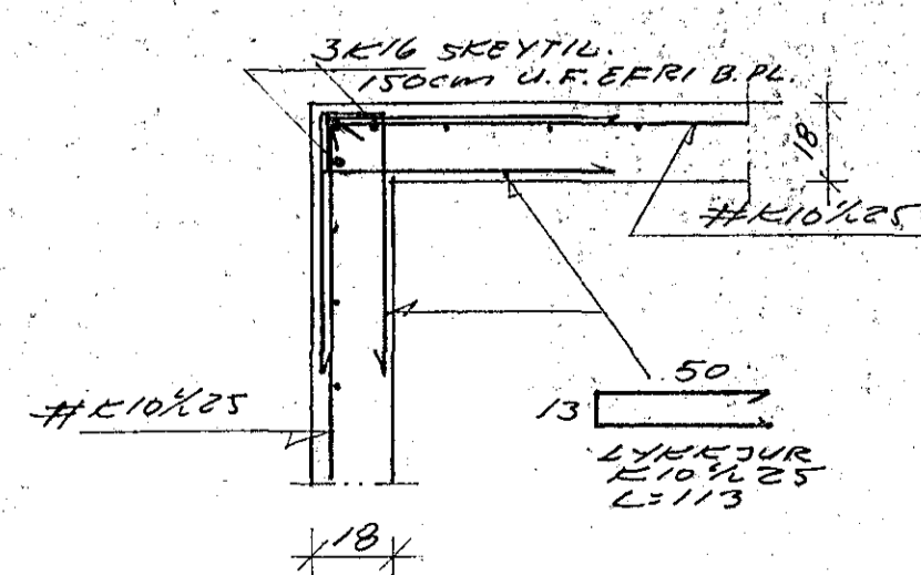
DEILI A2 1:20
