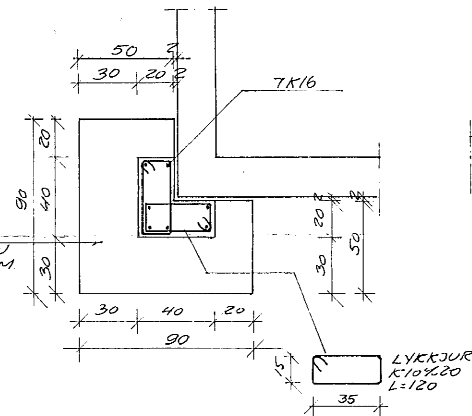
U7 1:20
