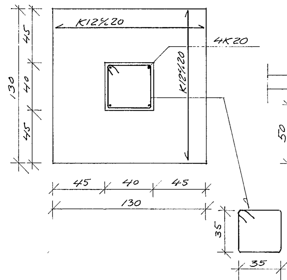
U5 1:20
