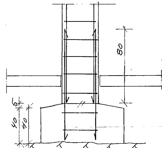
SNID d-d 1:20
