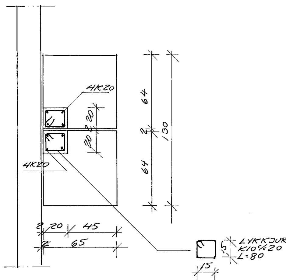
U9 1:20
