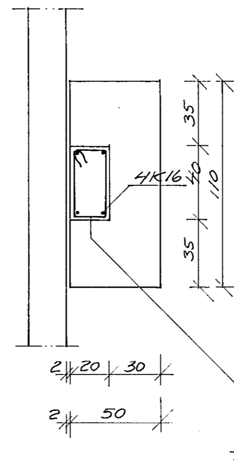
U3 1:20
