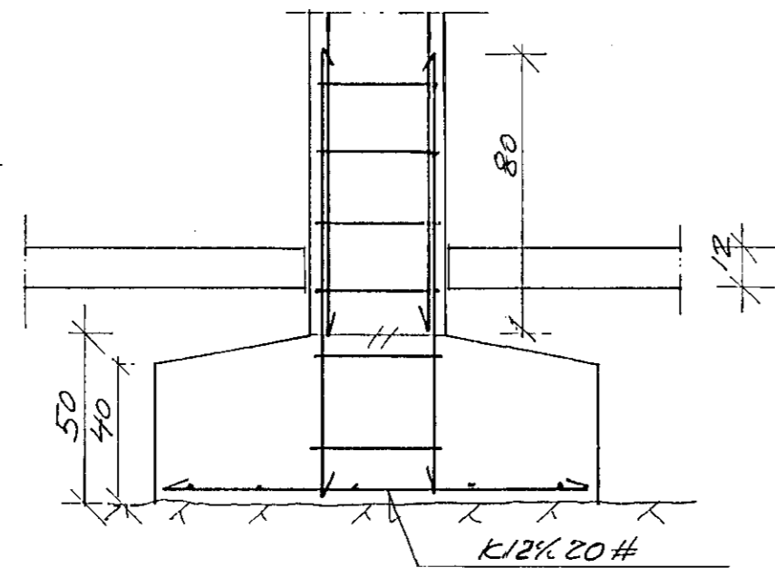
SNID a-a 1:20
