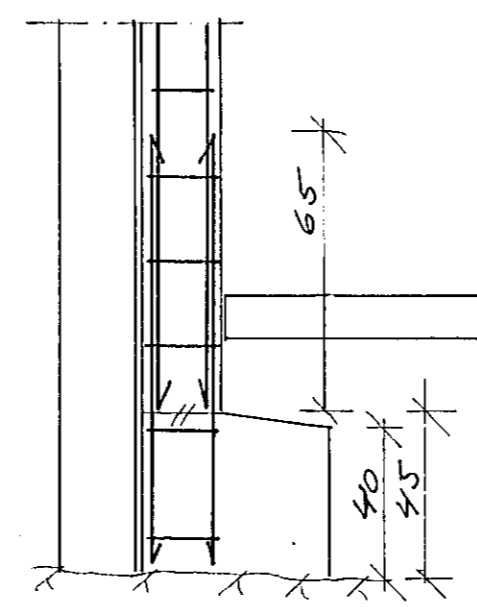
SNID b-b 1:20
