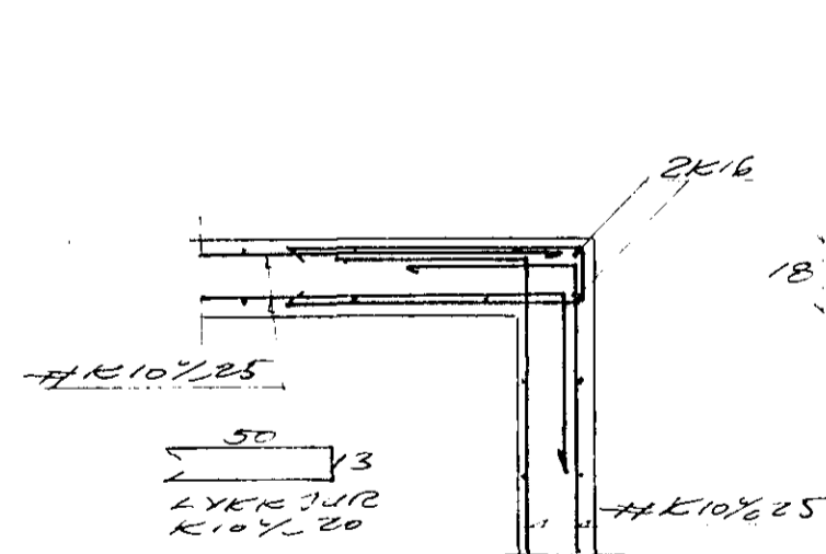
SNID P-P 1:20
