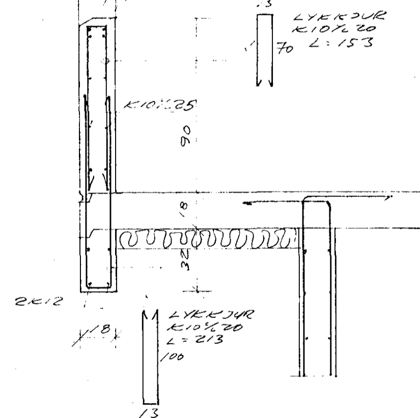
SNID U-U 1:20
